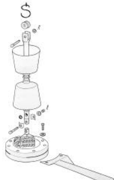
Montage samenstelling ventilator
