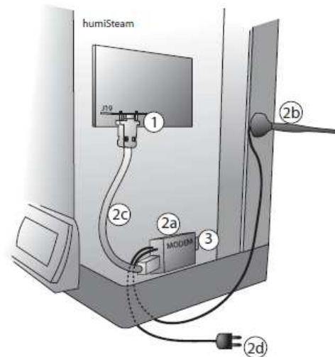
Fig. 5.c. (in het elektrische compartiment van de bevochtiger)
