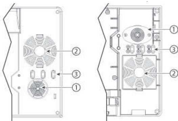
Modellen UE025 tot UE130 Zijaanzicht
