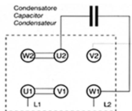
COLLEGAMENTO PER ROTAZIONE "A" CONNECTION FOR ROTATION "A" CONNEXION POUR ROTATION "A"
