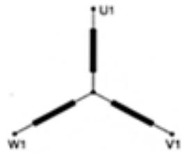
Collegamento Y Connection Y Connection Y
