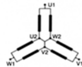
Alta velocità High speed Gran vitesse
