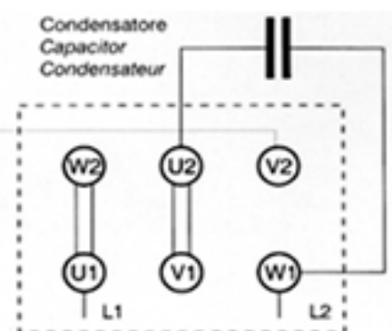
COLLEGAMENTO PER ROTAZIONE "B" CONNECTION FOR ROTATION "B" CONNEXION POUR ROTATION "B"
