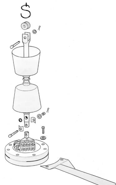
Montage samenstelling ventilator
