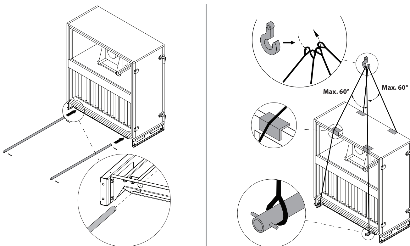
Fig. 14. Hijsen van afzonderlijke secties 1
