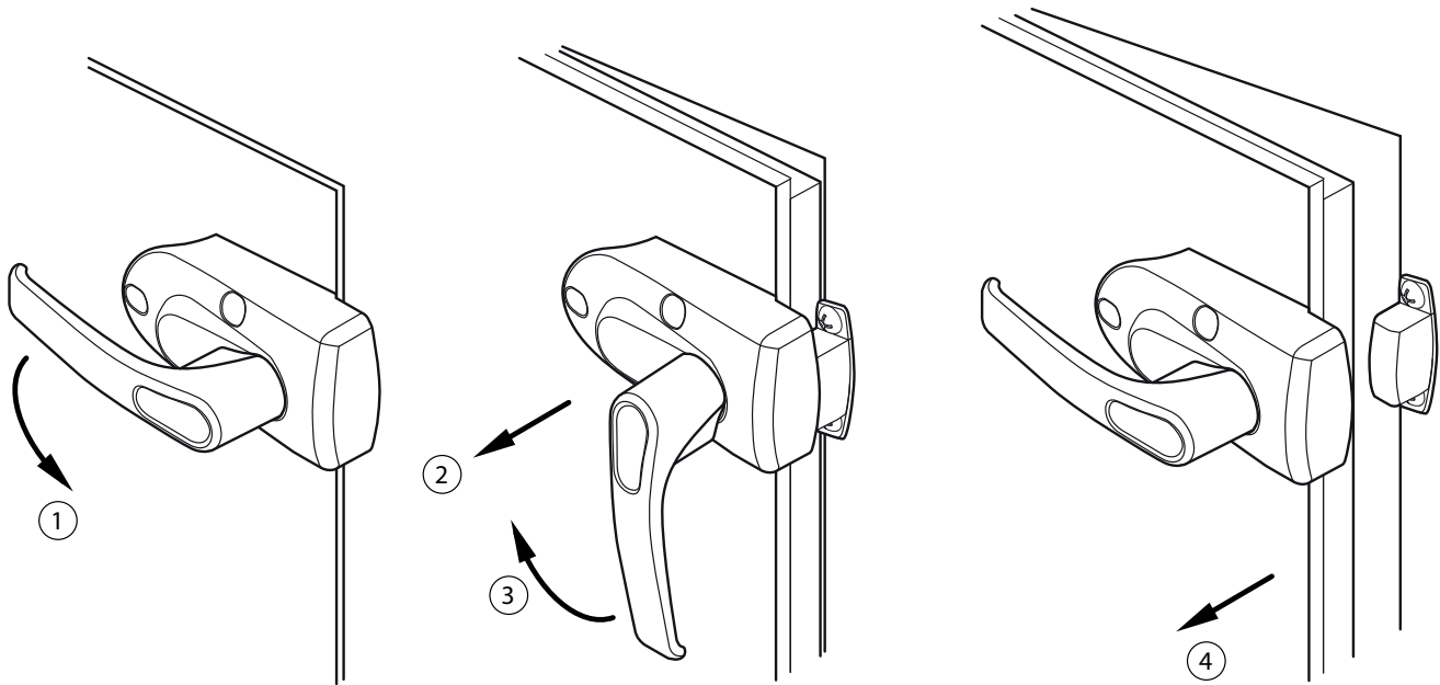
Fig. 19. Het openen van de deur
