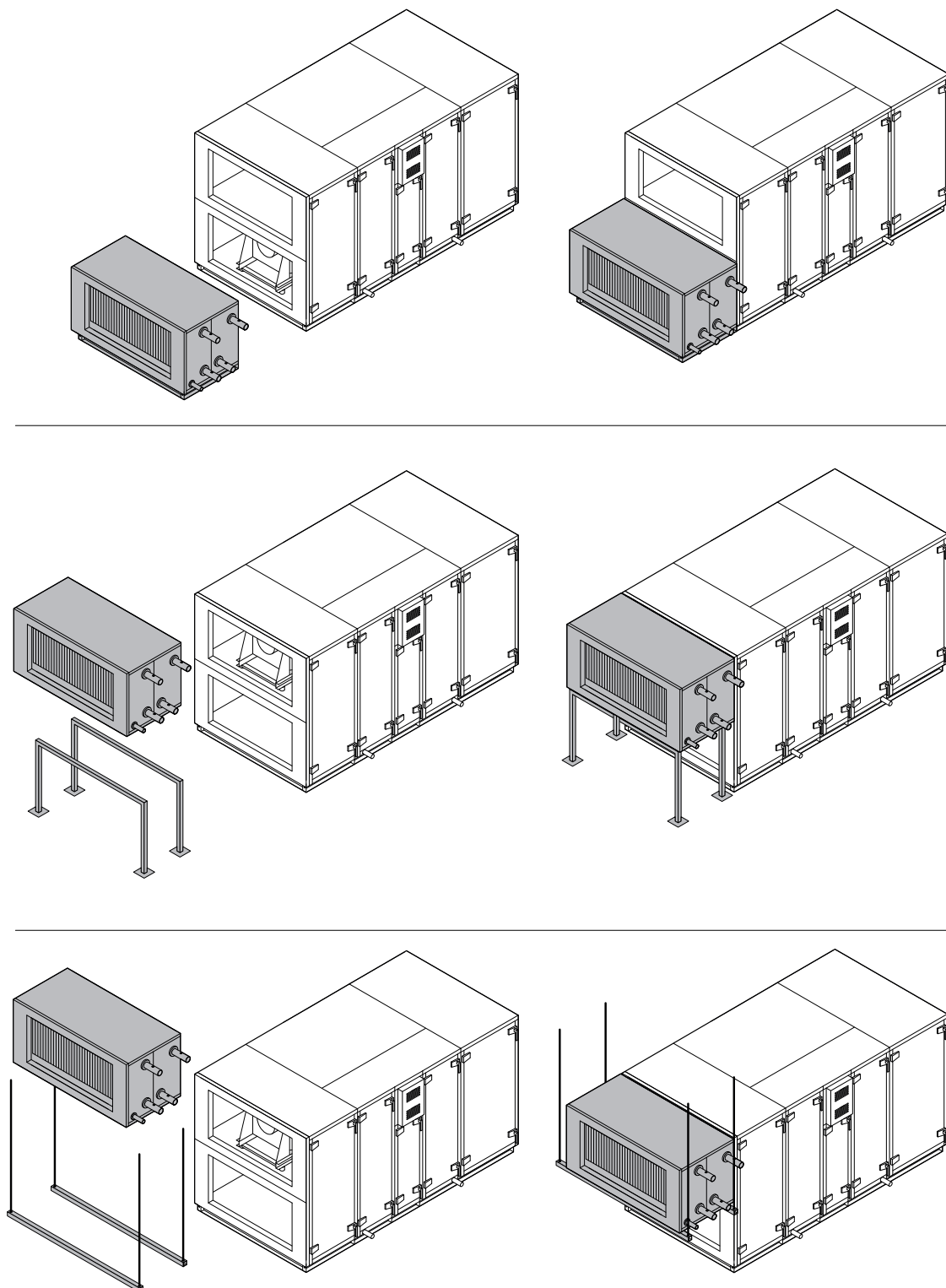
Fig. 24. Voorbeelden voor de installatie van verwarmings-/koelersecties
