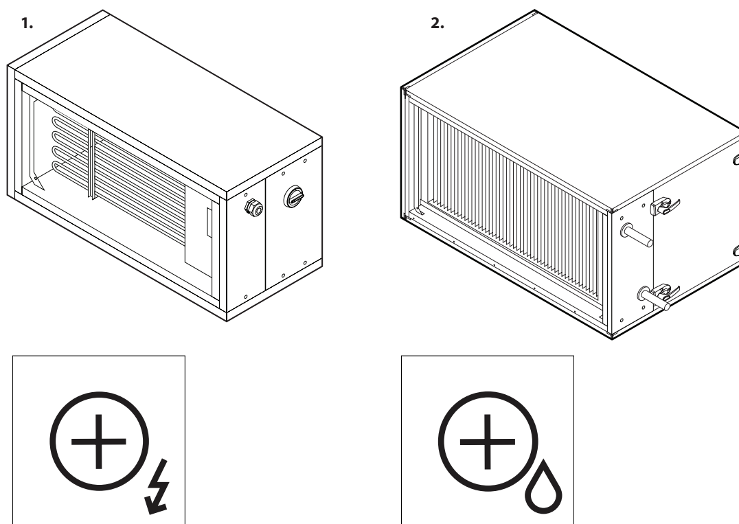
Fig. 8. Verwarmingssectie
