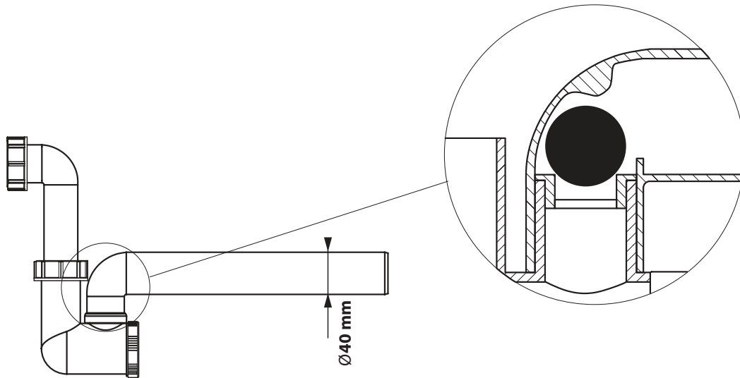
Fig. 29. Voorbeeld van een sifon met een eenrichtingsklep
