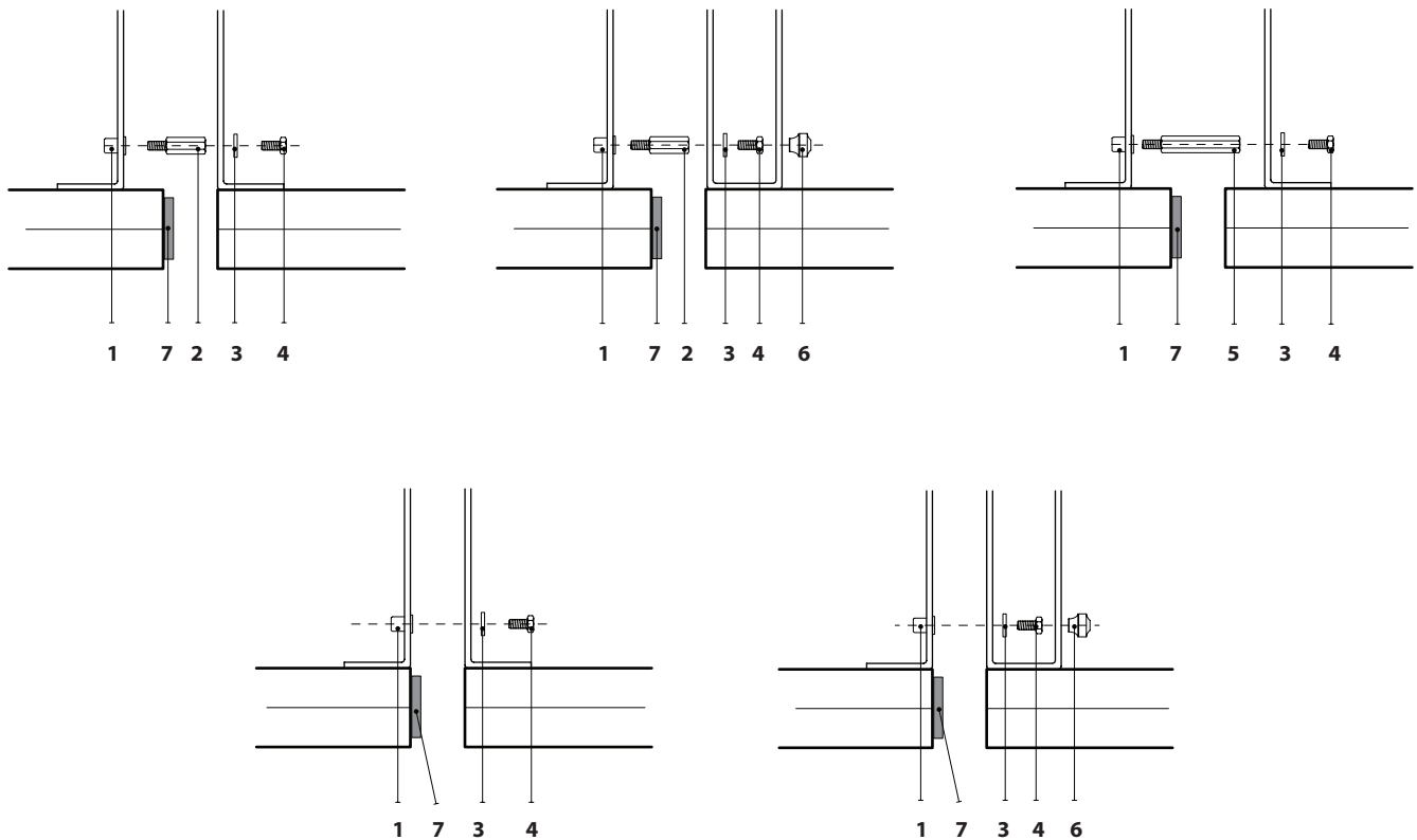
Fig. 22. Soorten interne sectieverbindingen
