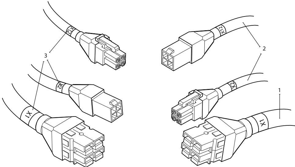
Fig. 48. Kabelverbindingen tussen secties
