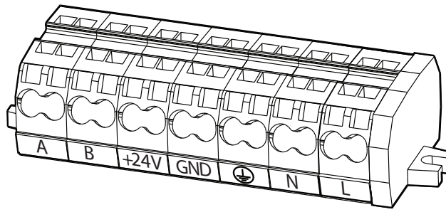
Fig. 44. Extra aansluitklemmenblok
