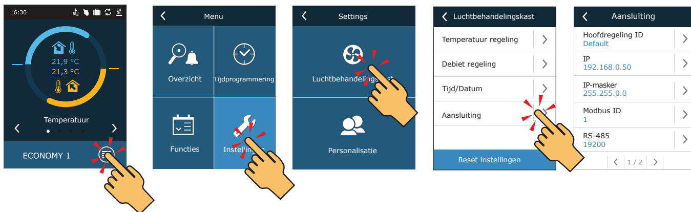
Fig. 50. Het bekijken en wijzigen van het IP-adres met een bedieningspaneel
