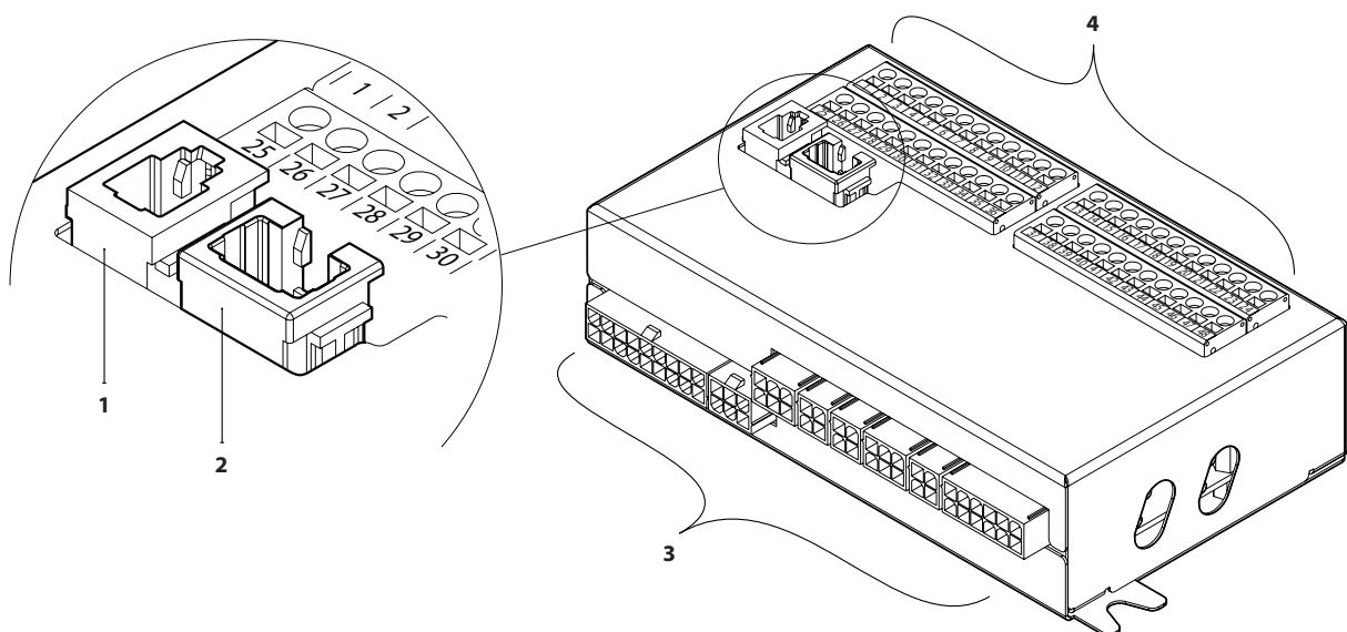
Fig. 38. Hoofdpaneel van het C5-bedieningspaneel
