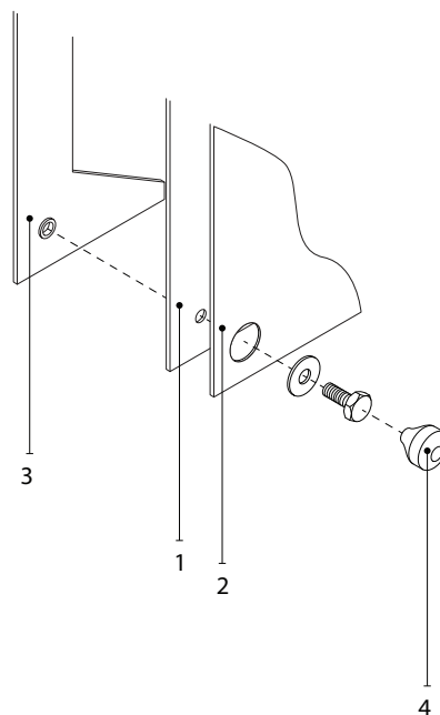
Fig. 23. Interne aansluiting in een ventilatorsectie
