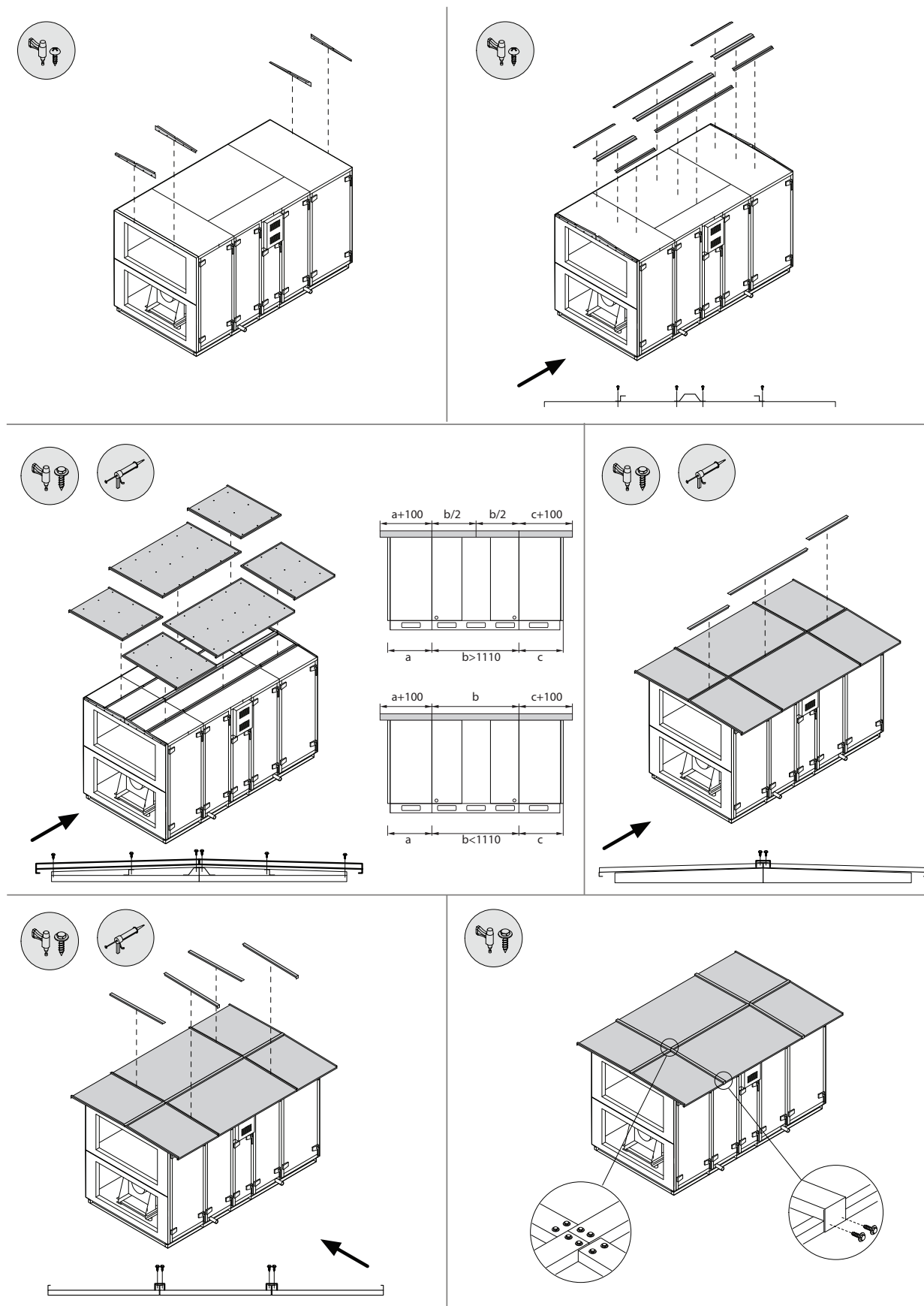
Fig. 34. Installatie van een afzonderlijk besteld beschermend dak 1
