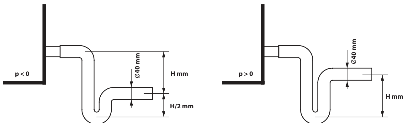
Fig. 28. Installatie van een sifon zonder eenrichtingsklep
