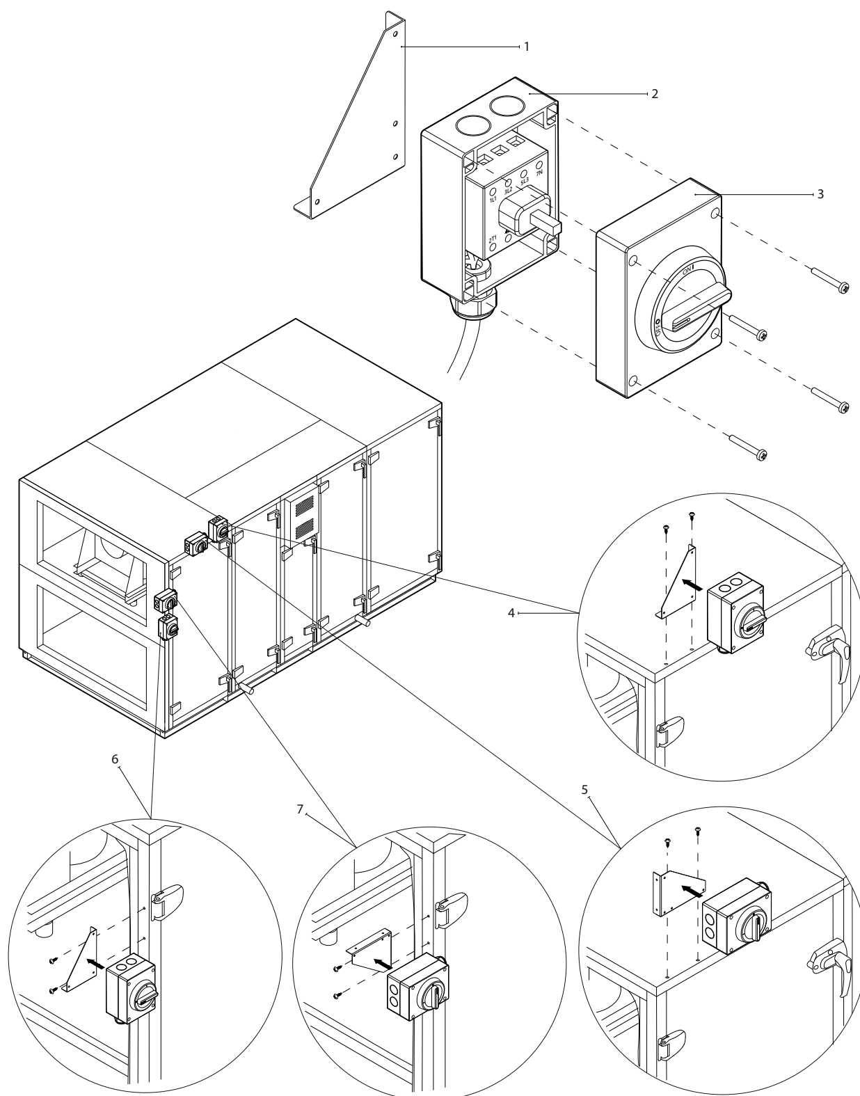
Fig. 35. Hoofdstroomonderbreker en montagevoorbeelden
