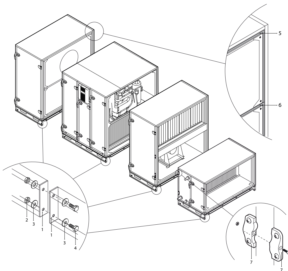
Fig. 21. Externe aansluiting en afdichting van secties
