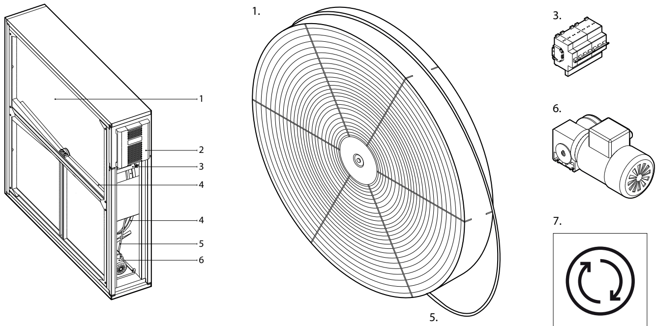
Fig. 3. Sectie Roterende Recuperator
