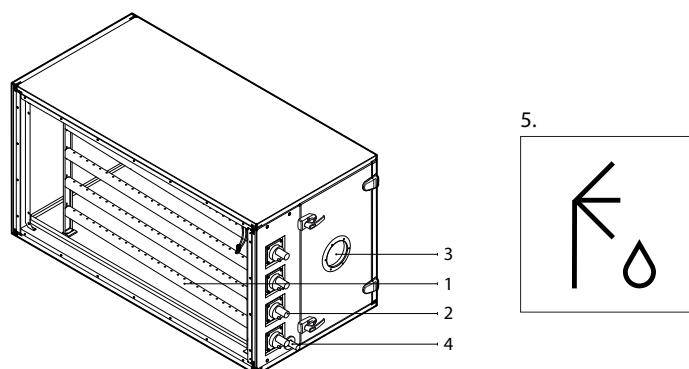
Fig. 11. Luchtbevochtiger
