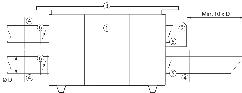
Afb. 33. Accessoires voor kasten die buiten worden geïnstalleerd
