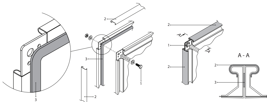
Fig. 31. Voorbeeld voor het bevestigen en afdichten van een flenskanaalverbinding 1 – schroef, 2 – C-profiel voor het aansluiten van flenzen, 3 – zelfklevende pakking
