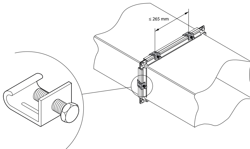
Fig. 32. Voorbeeld van kanaalaansluiting met universele klemverbindingen
