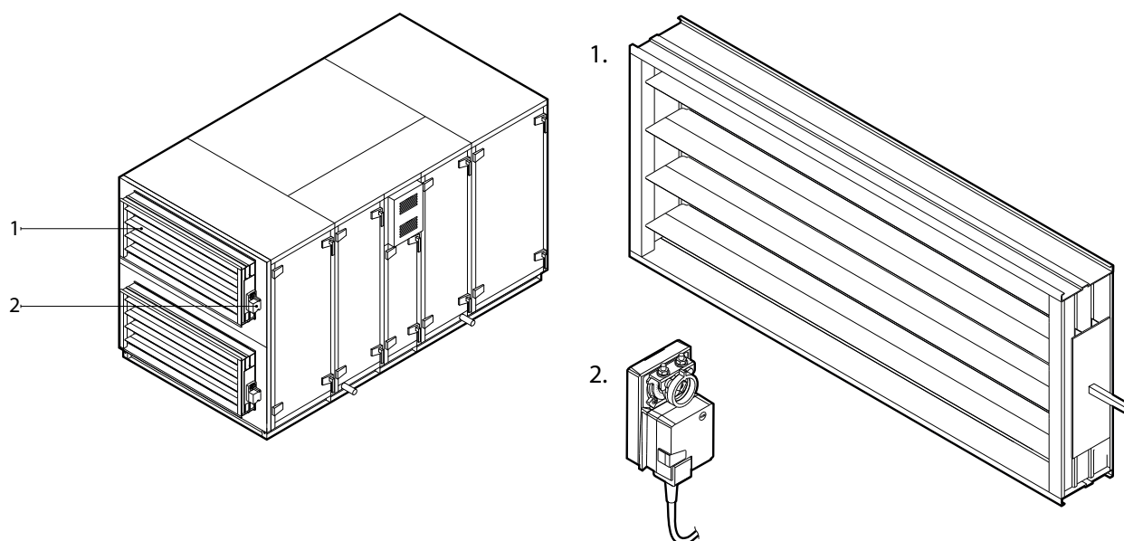
Fig. 9. Luchtafsluitende kleppen
