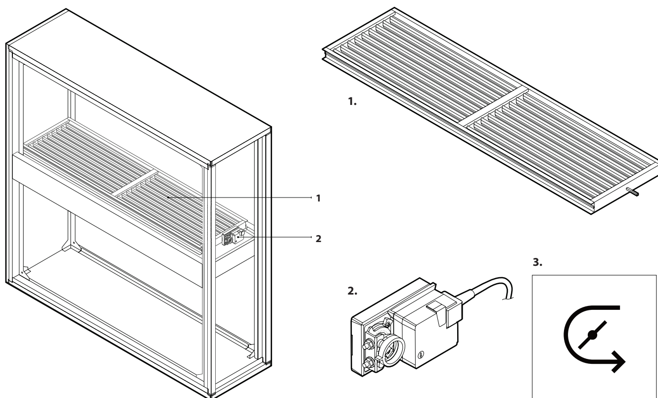
Fig. 6. Recirculatiesectie
