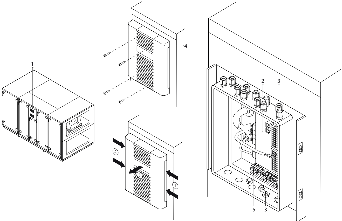
Fig. 37. Automatiseringskast
