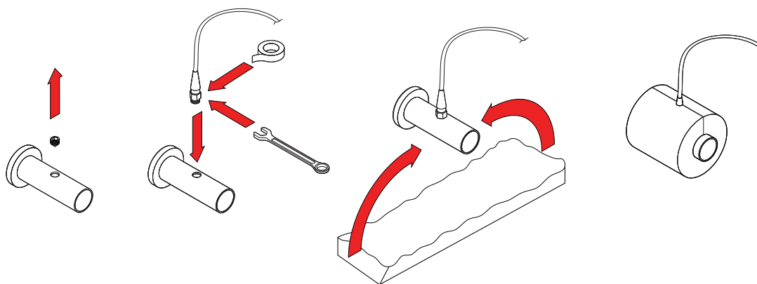
Fig. 27. Installatie van een retourwatertemperatuursensor met schroefdraad 1
