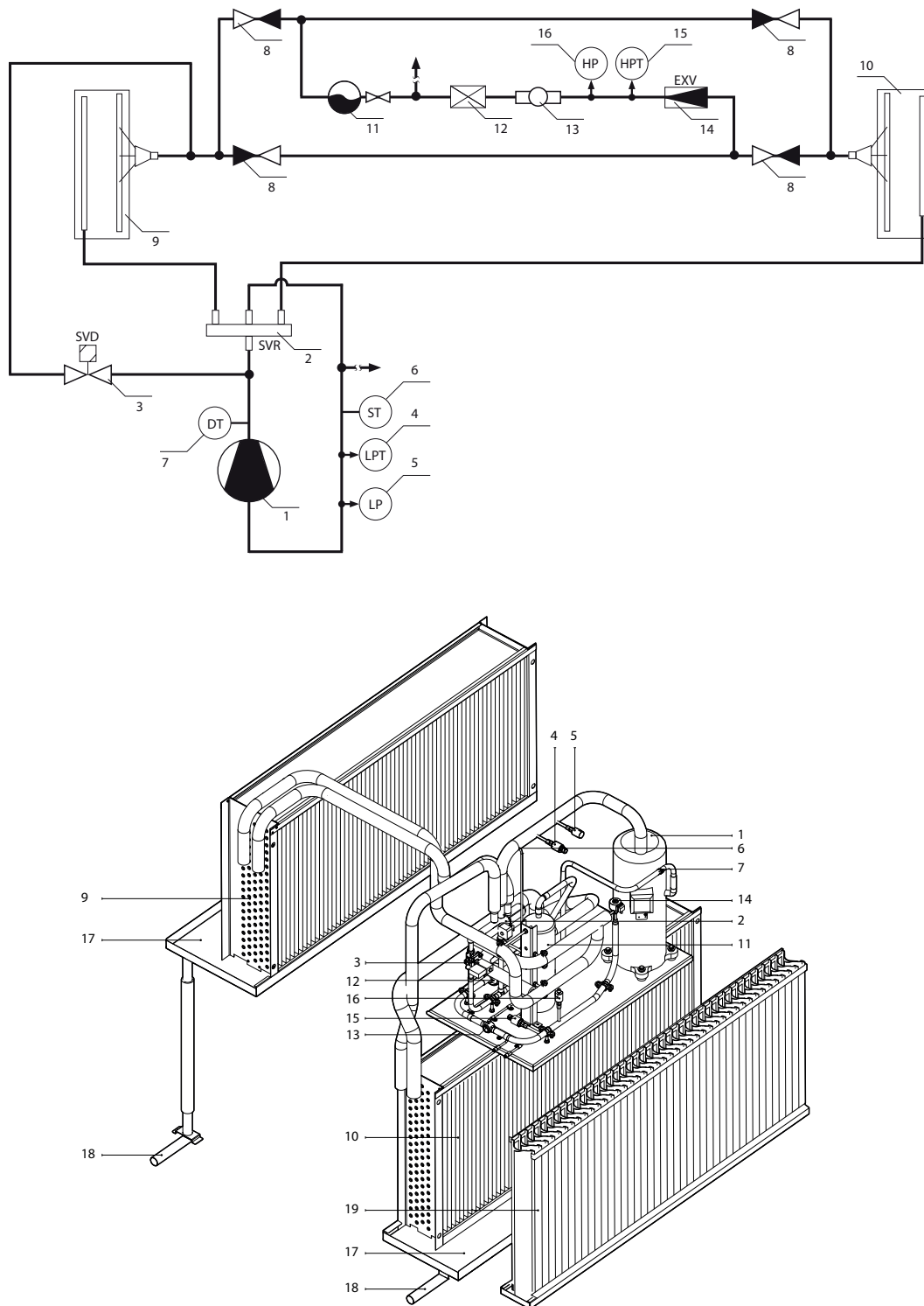
Fig. 4. Hydraulisch schakelschema en onderdelen van de warmtepomp
