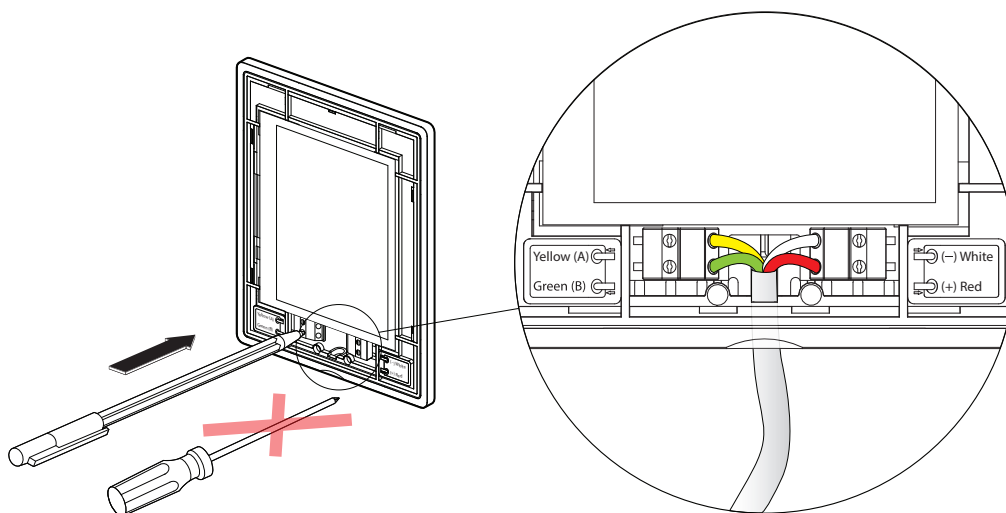
Fig. 47. Bedrading bedieningspaneel
