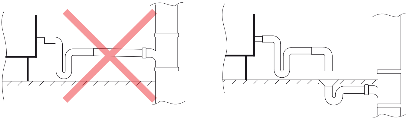
Fig. 30. Aansluiting van de condensaatafvoer op de riolering
