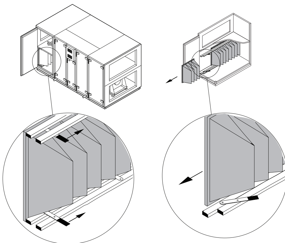
Fig. 53. Filterkleminrichting
