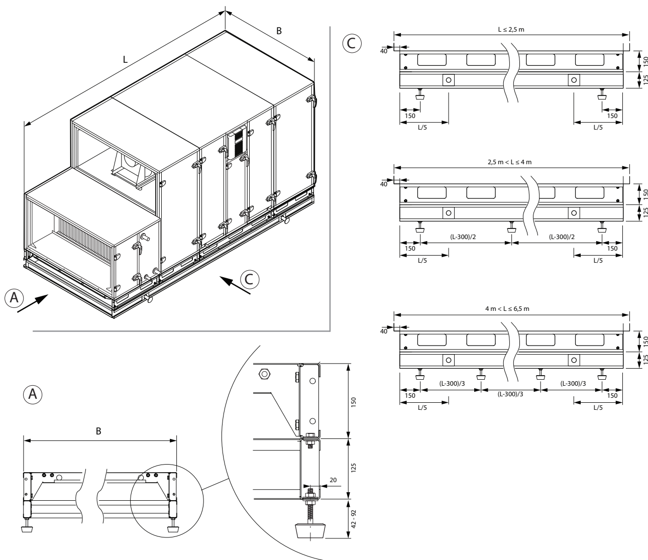
Fig. 16. Afmetingen van het versterkt montageframe
