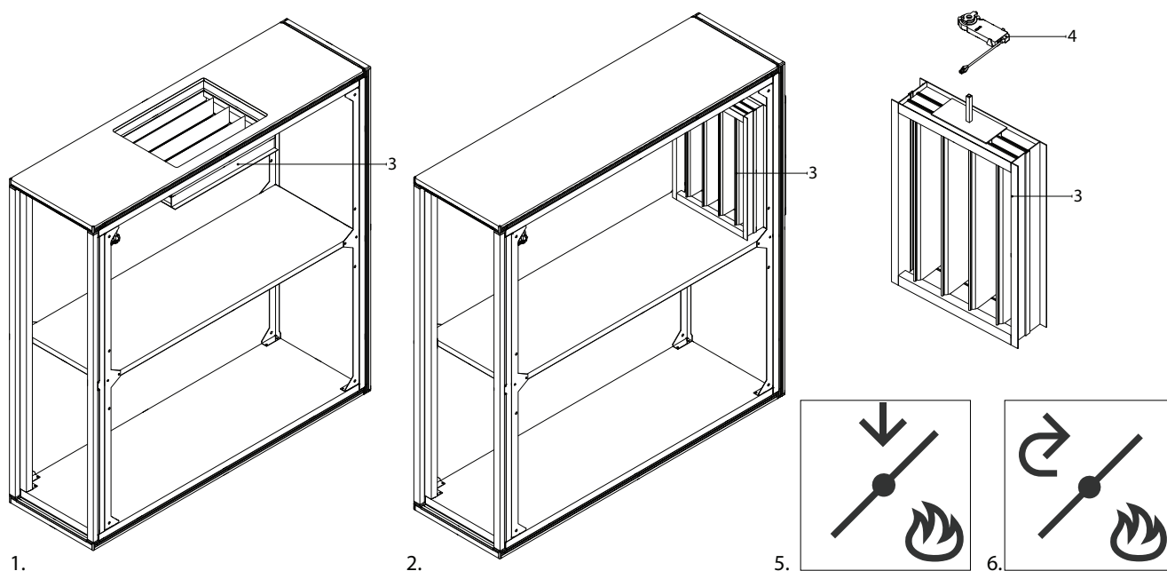
Fig. 12. Rookafvoersectie
