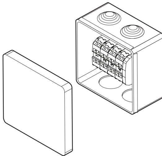
Fig. 49. Aftakdoos PD1
