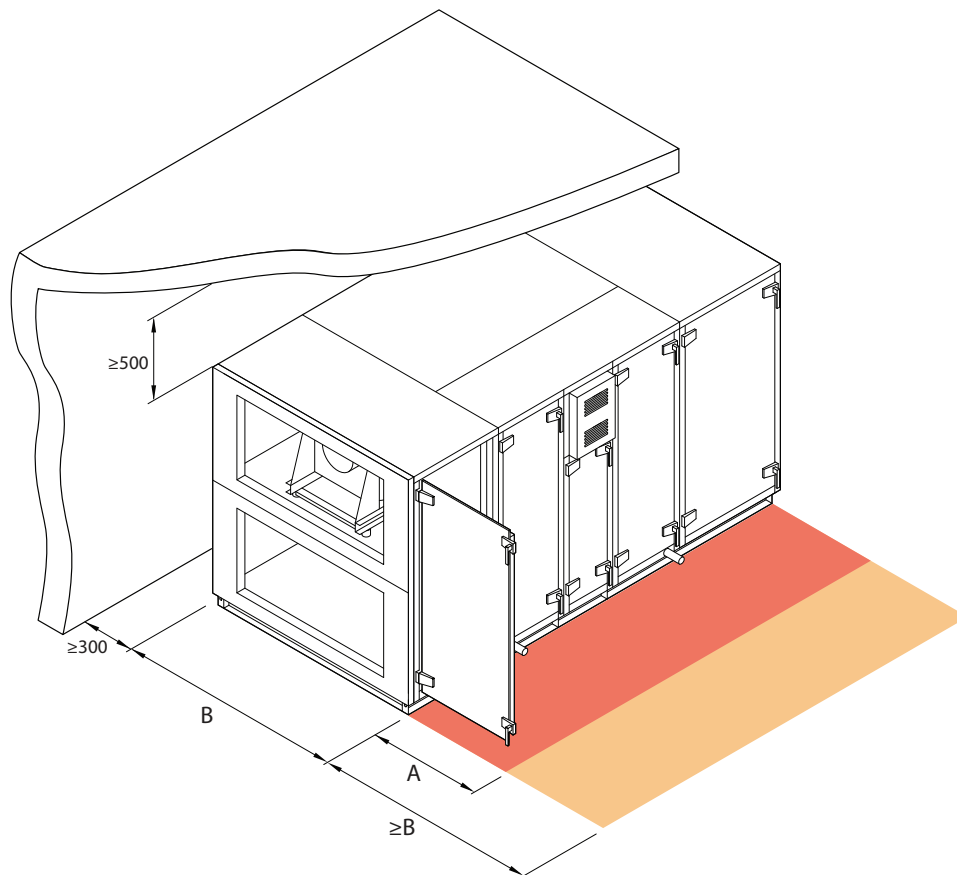
Fig. 18. Kastinspectiegebied
