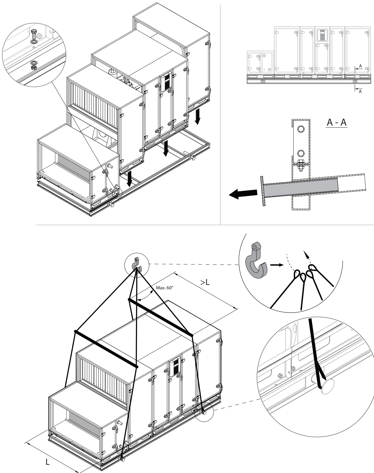
Fig. 15. LBK volledig gemonteerd op een versterkt montageframe tillen 1
