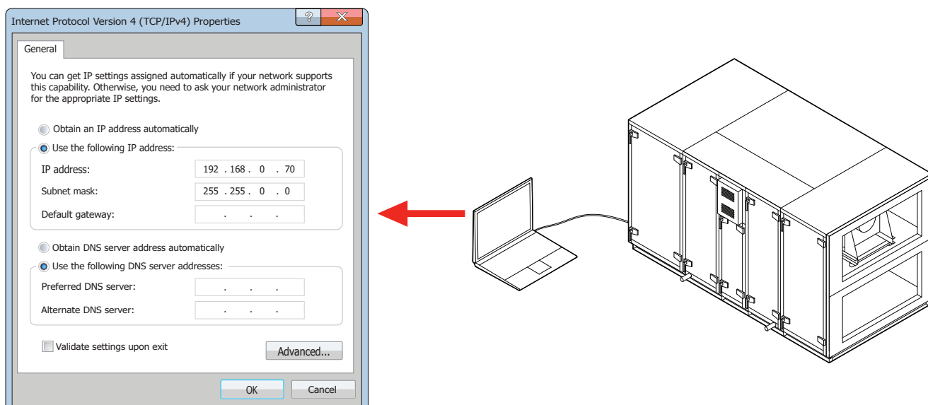
Fig. 51. Computernetwerkinstellingen voor directe aansluiting op de kast
