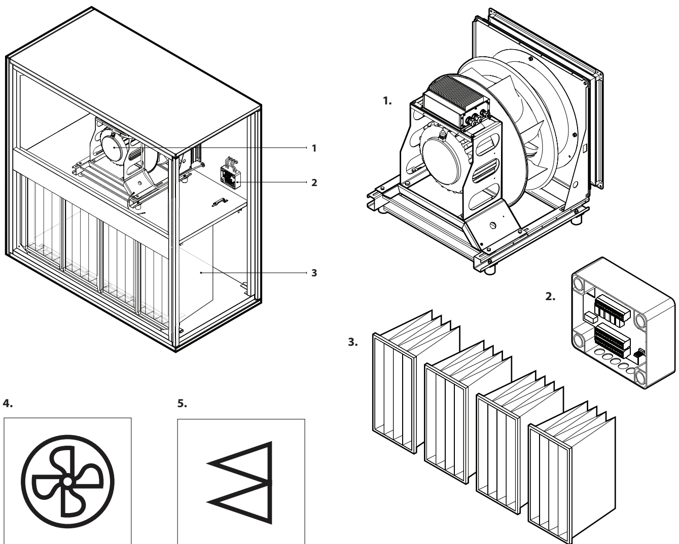
Fig. 1. Filterventilatorsectie
