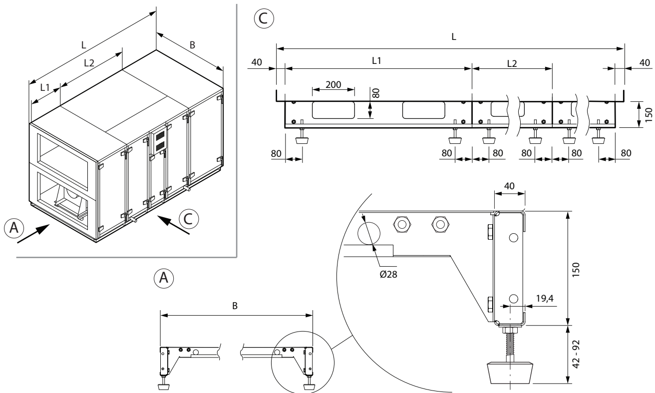
Fig. 17. Inbouwframe met verstelbare poten
