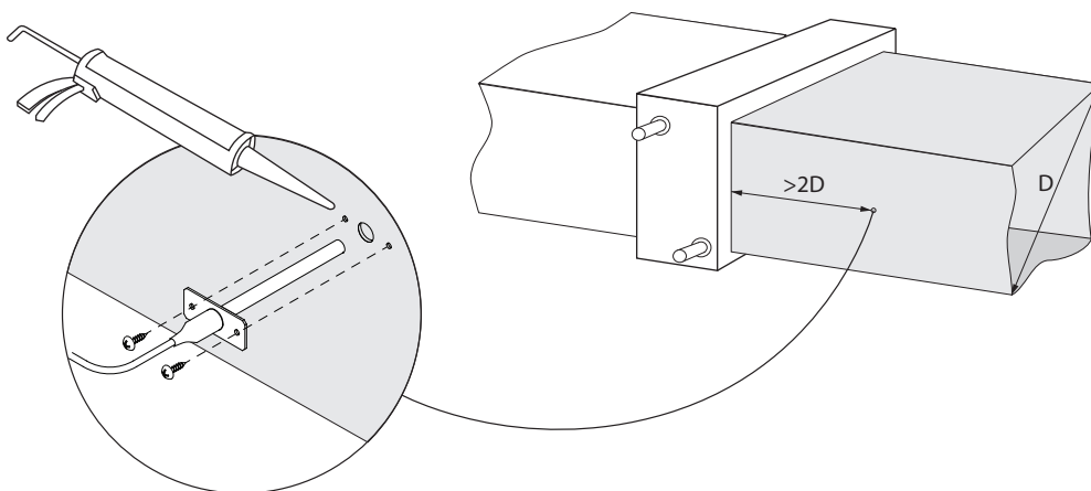
Fig. 43. Installatie van een toevoerluchttemperatuursensor
