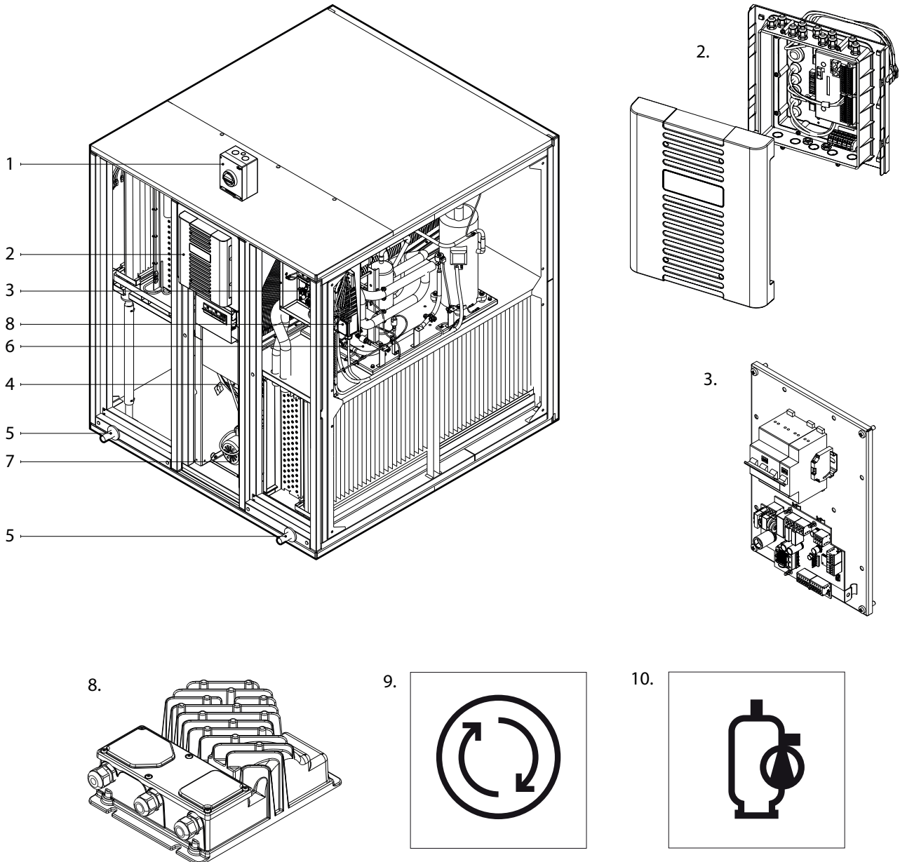
Fig. 2. Warmtepompsectie
