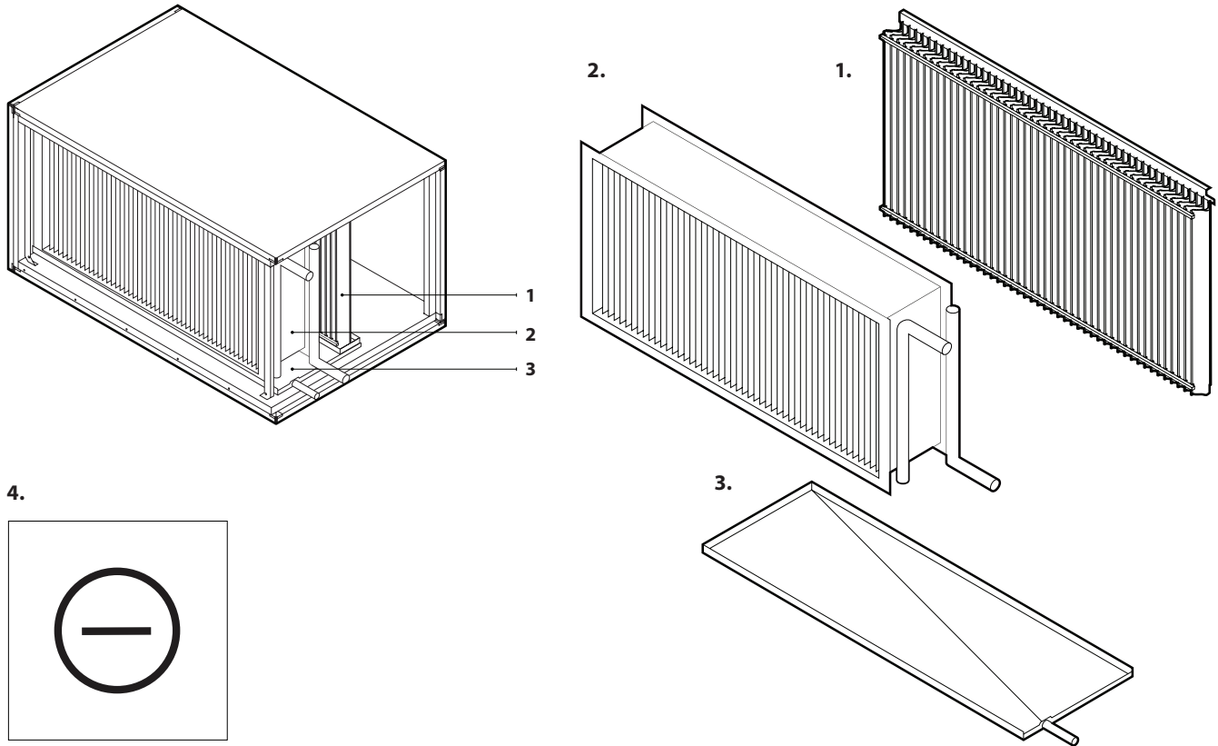
Fig. 7. Koelersectie
