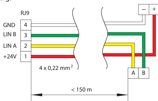
Fig. 46. Bedieningspaneel bedradingsschema
