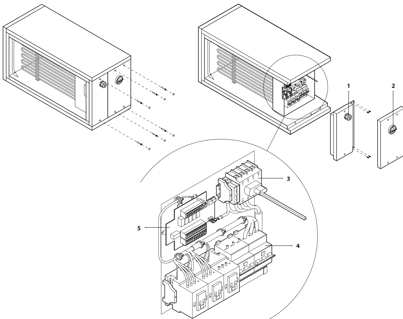
Fig. 36. Hoofdstroomonderbreker in een elektrisch verwarmingssectie
