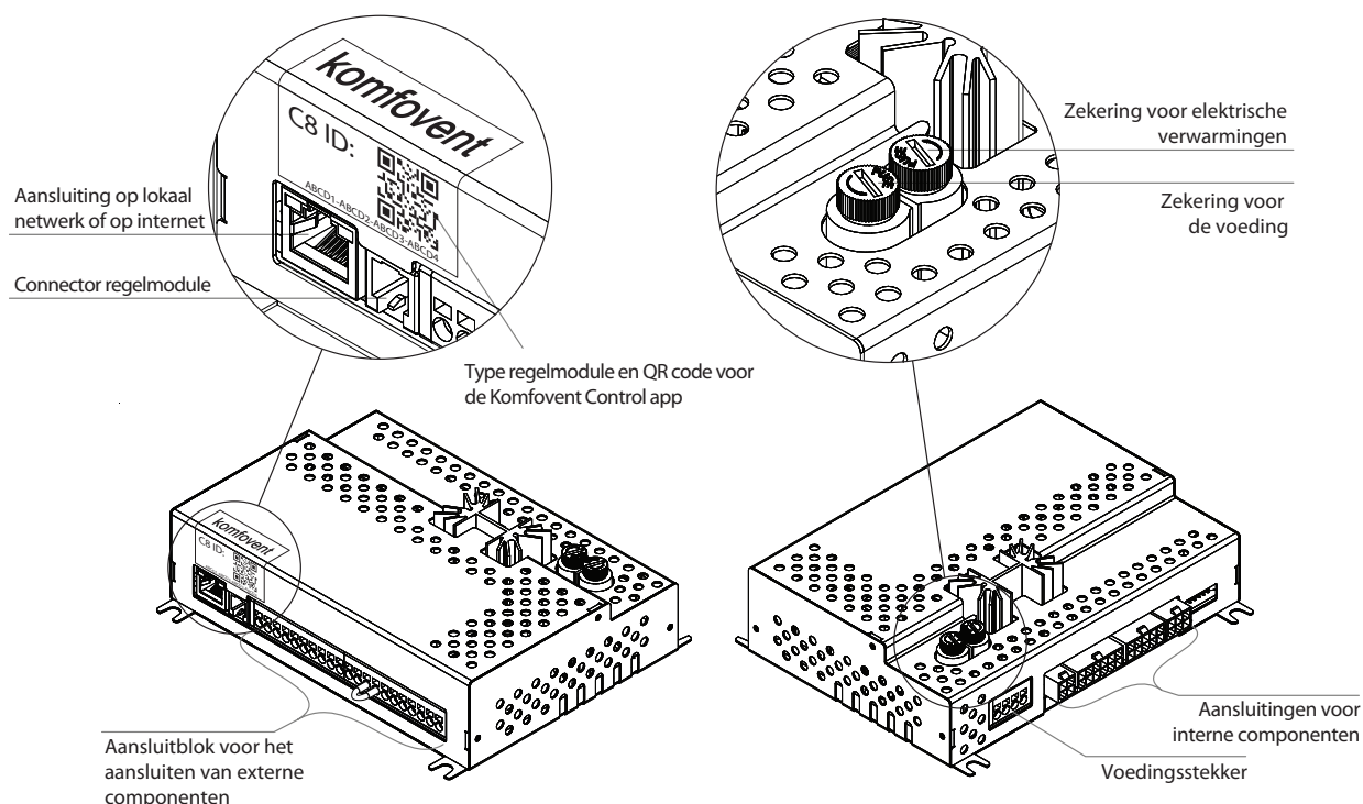
Afb. 10. C8 hoofdregelmodule
