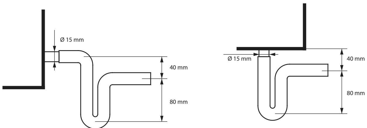
Afb. 9a. Installatie van de sifon zonder terugslagklep
