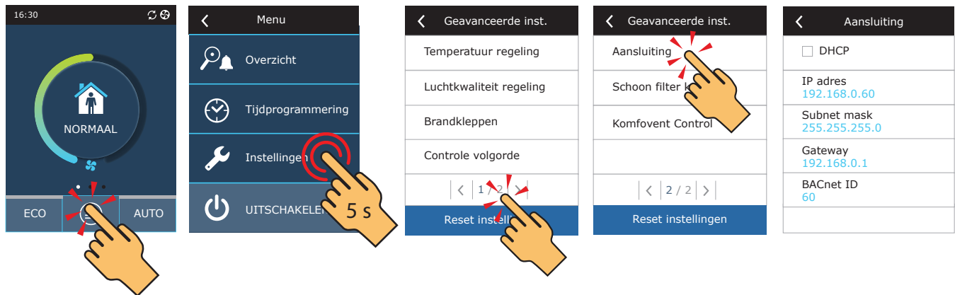
Afb. 16. Vind en wijzig het IP-adres van de luchtbehandelingskast op het regelpaneel
