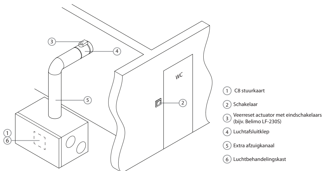
Afb. 7. Montagevoorbeeld van een extra luchtafzuigkanaal
