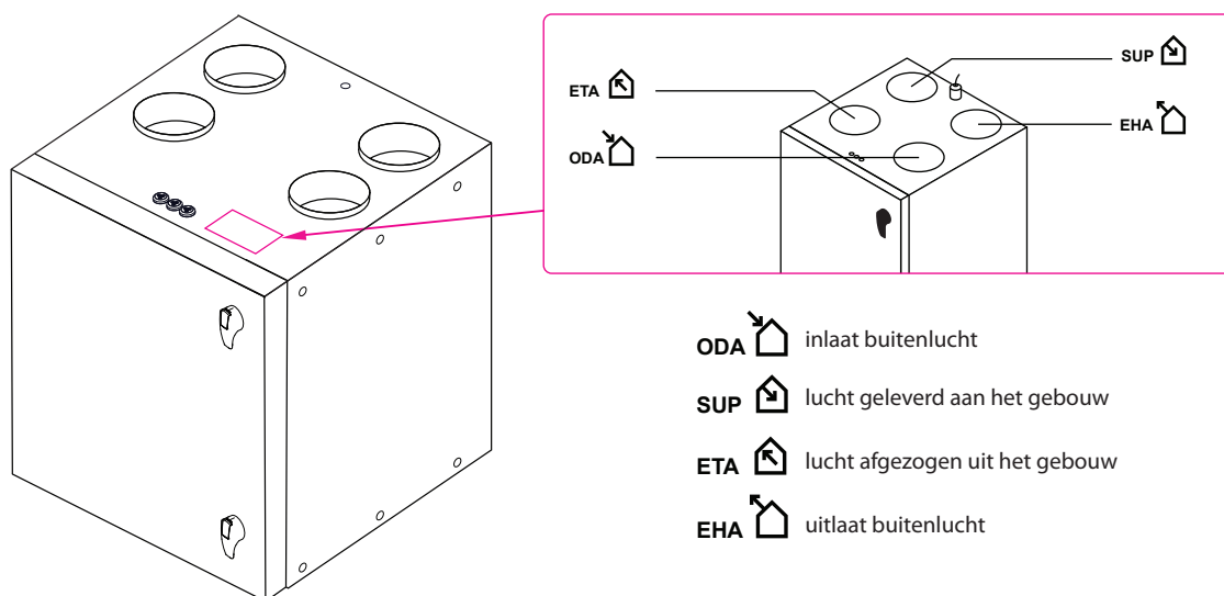
Afb. 6. Markering luchtkanaal
