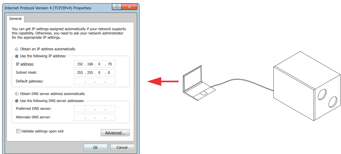
Afb. 17. Netwerkinstellingen van de computer voor een rechtstreekse verbinding met de kast
