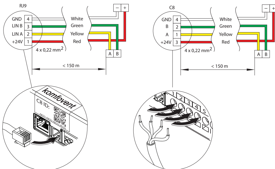
Afb. 14. Bedradingschema kabel regelpaneel
