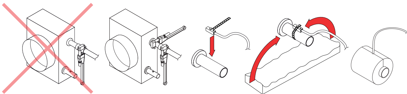
Afb. 8. Het aansluiten van de waterslangen op de verwarming/koeler en het installeren van de watertempatuursensor
