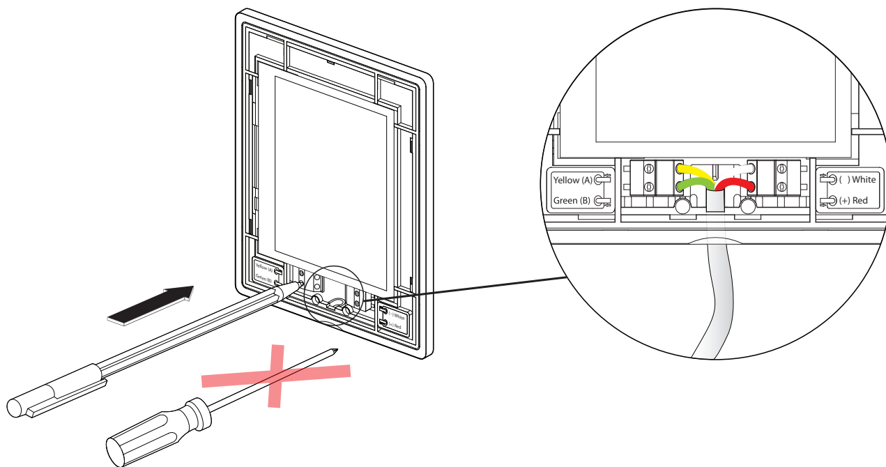
Afb. 15. Kabel aansluiten op het regelpaneel
