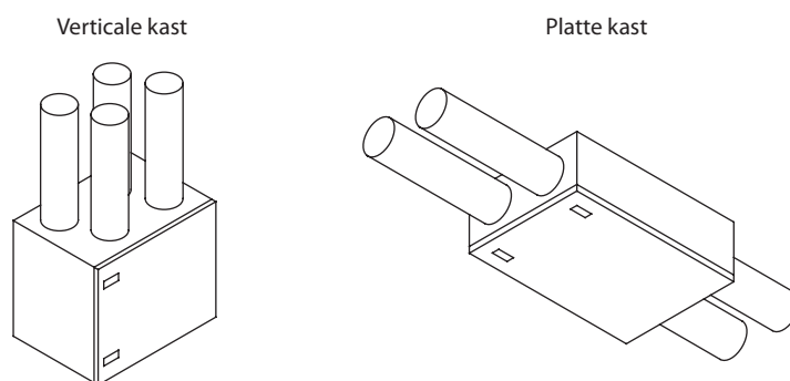
Afb. 1. Classificatie van kasten o.b.v. het type kanaalaansluiting
