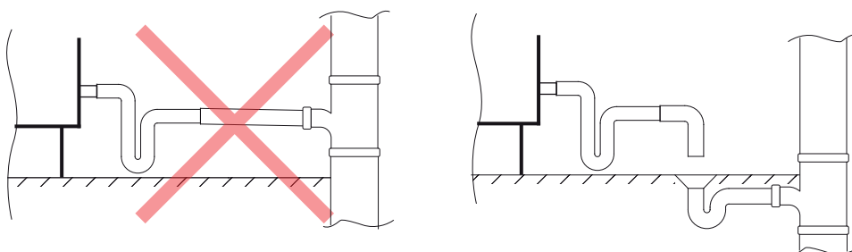
Afb. 9b. Aansluiting van de condens afvoer op de riolering
