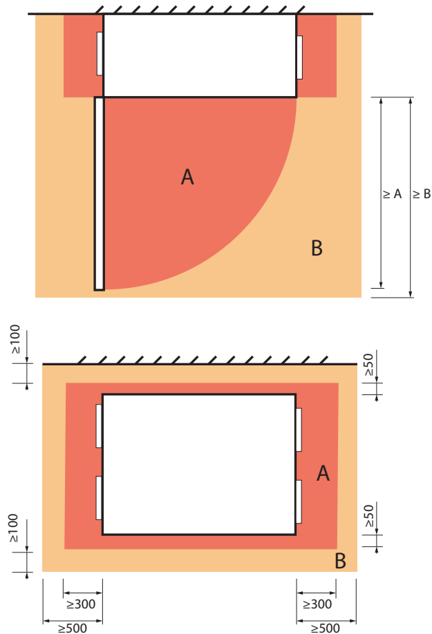
Afb. 5. Minimale ruimte voor onderhoud
