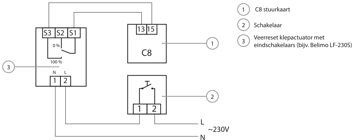
Afb. 13. Voorbeeld van een "Override" ventilatiemodus bij gebruik van extra luchtafzuiging. met een gemotoriseerde afsluitklep (zie afb. 7)
