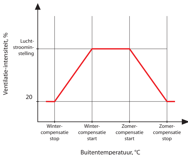
Fig. 2 OCV-functiebediening
