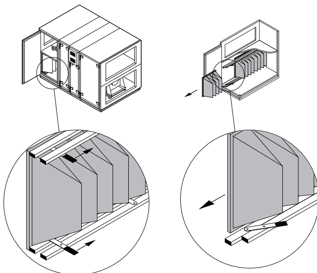
Fig. 4 Filterkleminrichting
