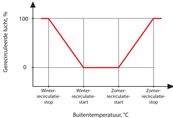
Fig. 3 REC-functiebediening
