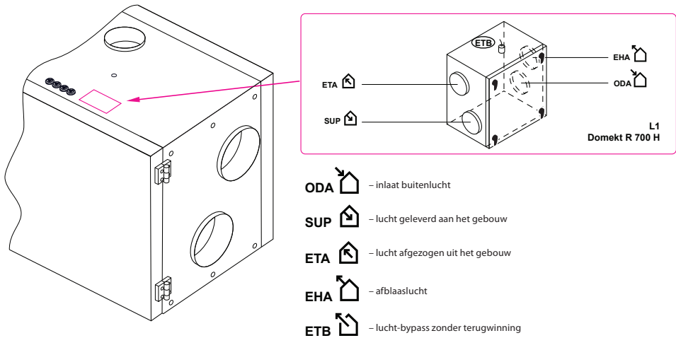
Afb. 9. Markering luchtkanaal
