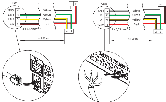
Afb. 17. Bedradingsschema kabel regelpaneel
