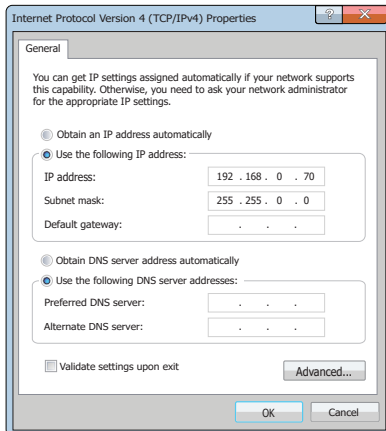
Afb. 20. Netwerkinstellingen van de computer voor een rechtstreekse verbinding met de kast
