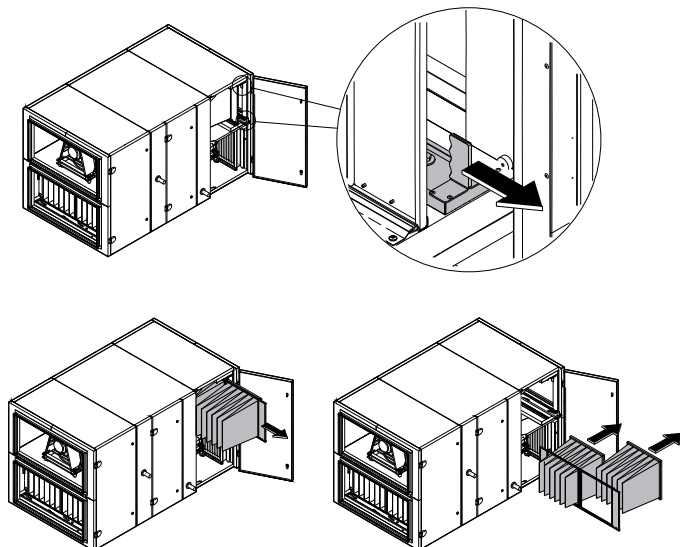
Fig. 3. Filterkleminrichting
