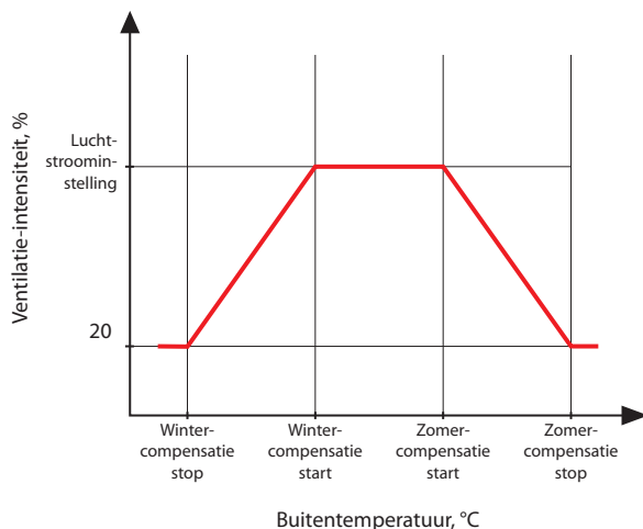
Fig. 1. OCV-functiebediening
