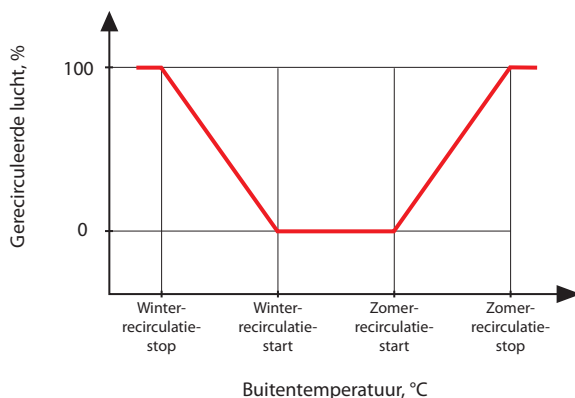
Fig. 2. REC-functiebediening
