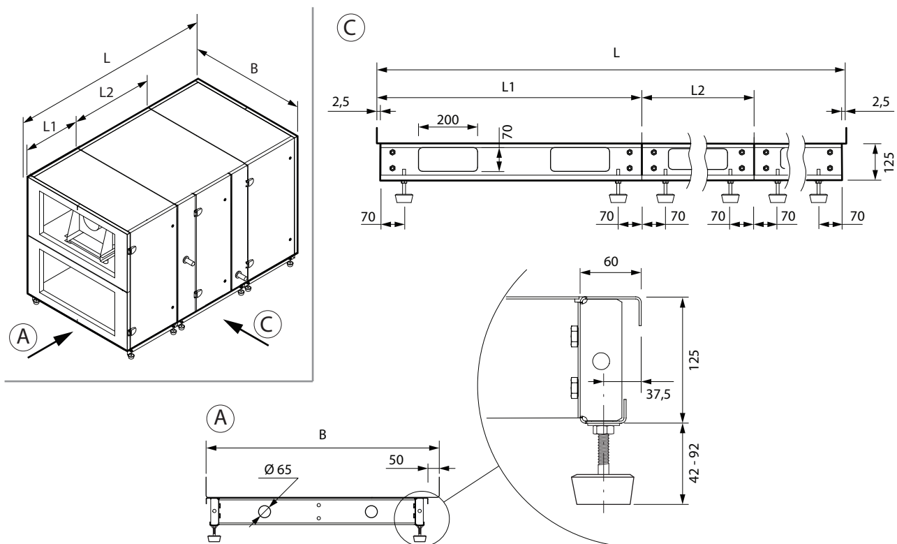
Fig. 13. Inbouwframe met verstelbare poten
