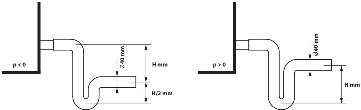
Fig. 21. Installatie van een sifon zonder eenrichtingsklep
