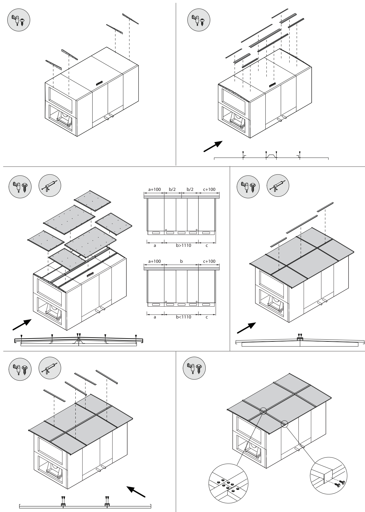
Fig. 27. Installatie van een afzonderlijk besteld beschermend dak 1
