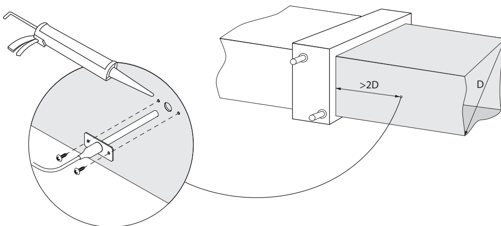
Fig. 36. Installatie van een toevoerluchttemperatuursensor
