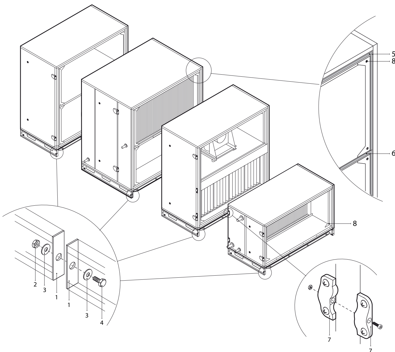
Fig. 16. Externe aansluiting en afdichting van secties
