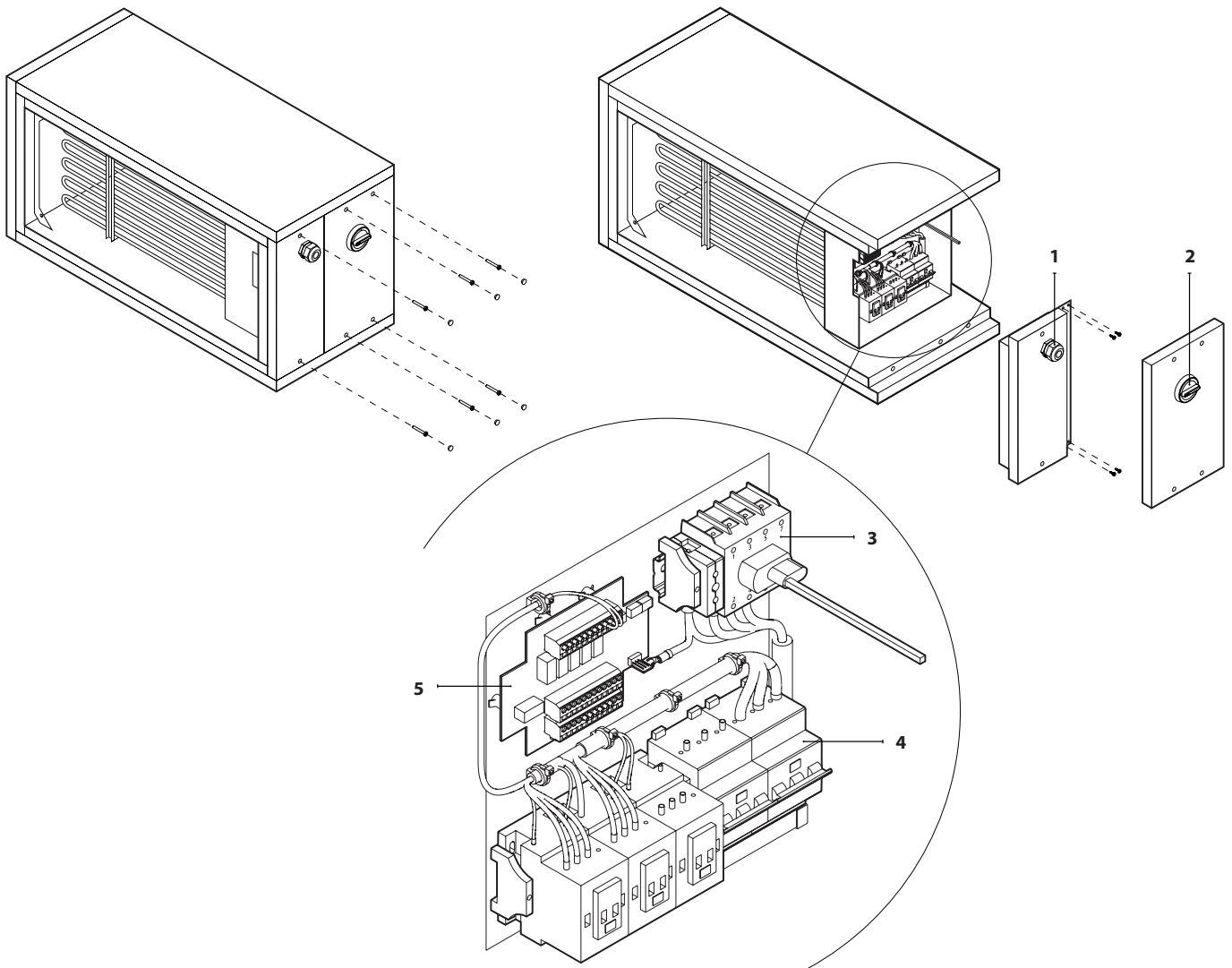
Fig. 29. Hoofdstroomonderbreker in een elektrisch verwarmingssectie
