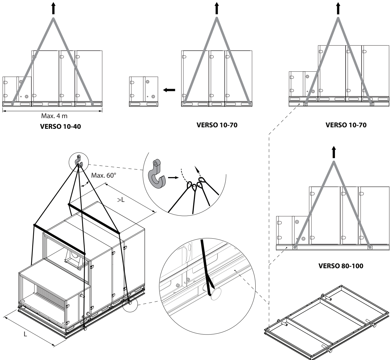
Fig. 12. LBK volledig gemonteerd op een versterkt montageframe tillen 1
