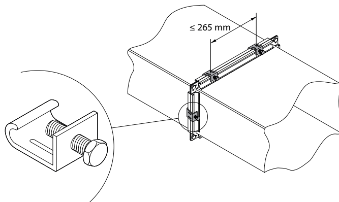
Fig. 25. Voorbeeld van kanaalaansluiting met universele klemverbanden
