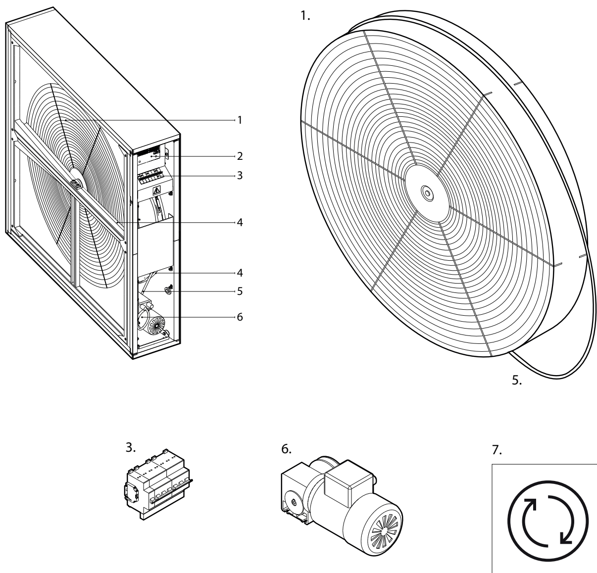
Fig. 3. Sectie Roterende Recuperator
