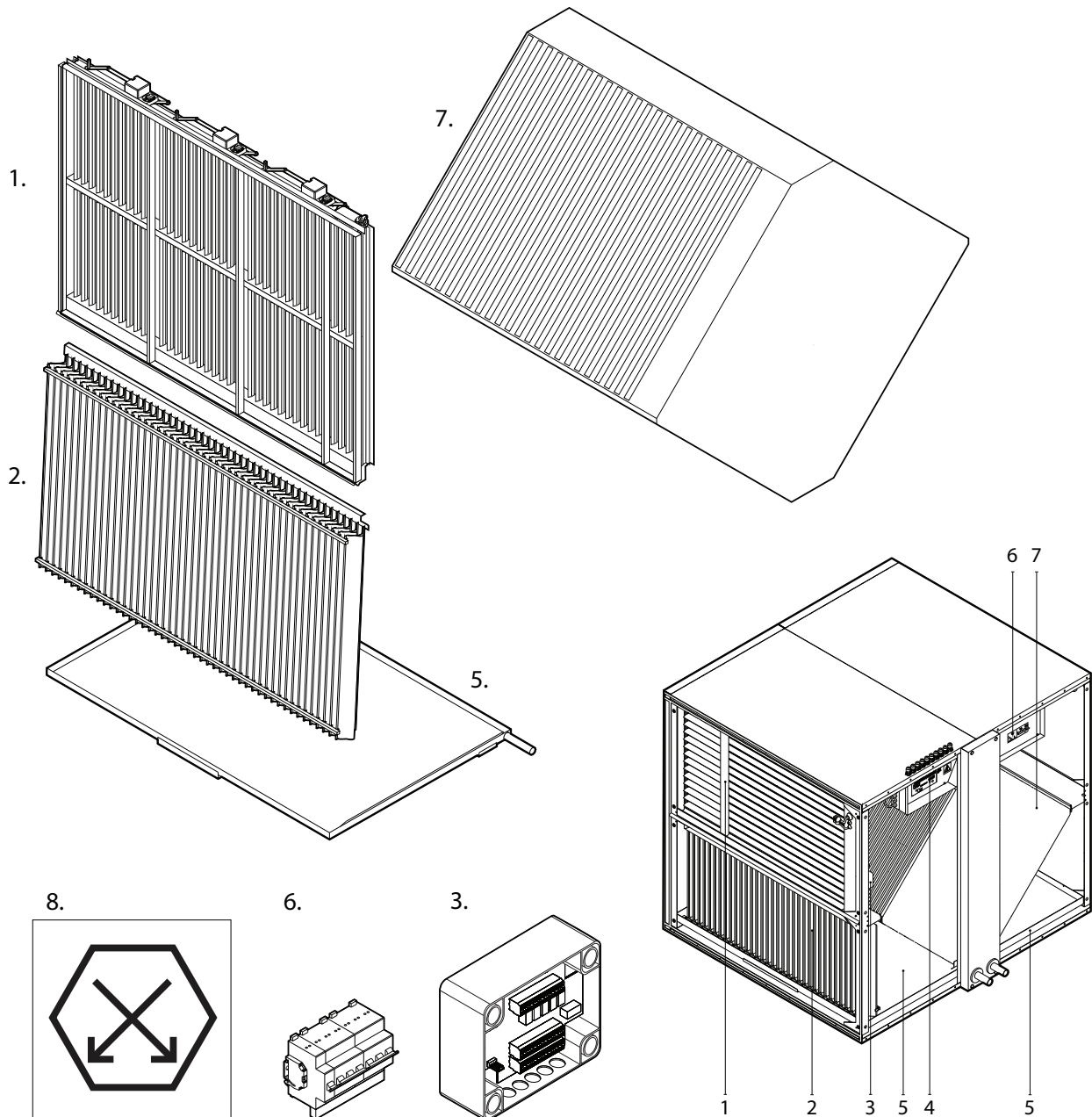
Fig. 2. Sectie Tegenstroomwarmtewisselaar (CF)
