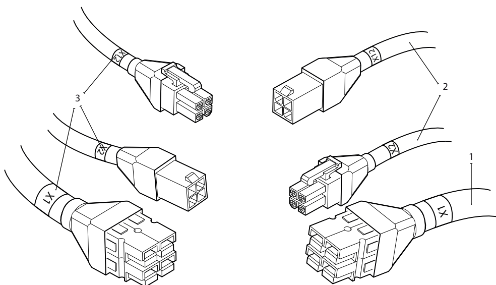
Fig. 39. Kabelverbindingen tussen secties
