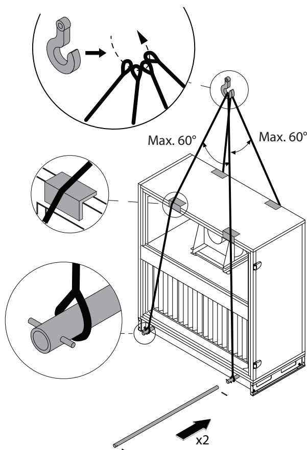
Fig. 11. Hijsen van afzonderlijke secties 1
