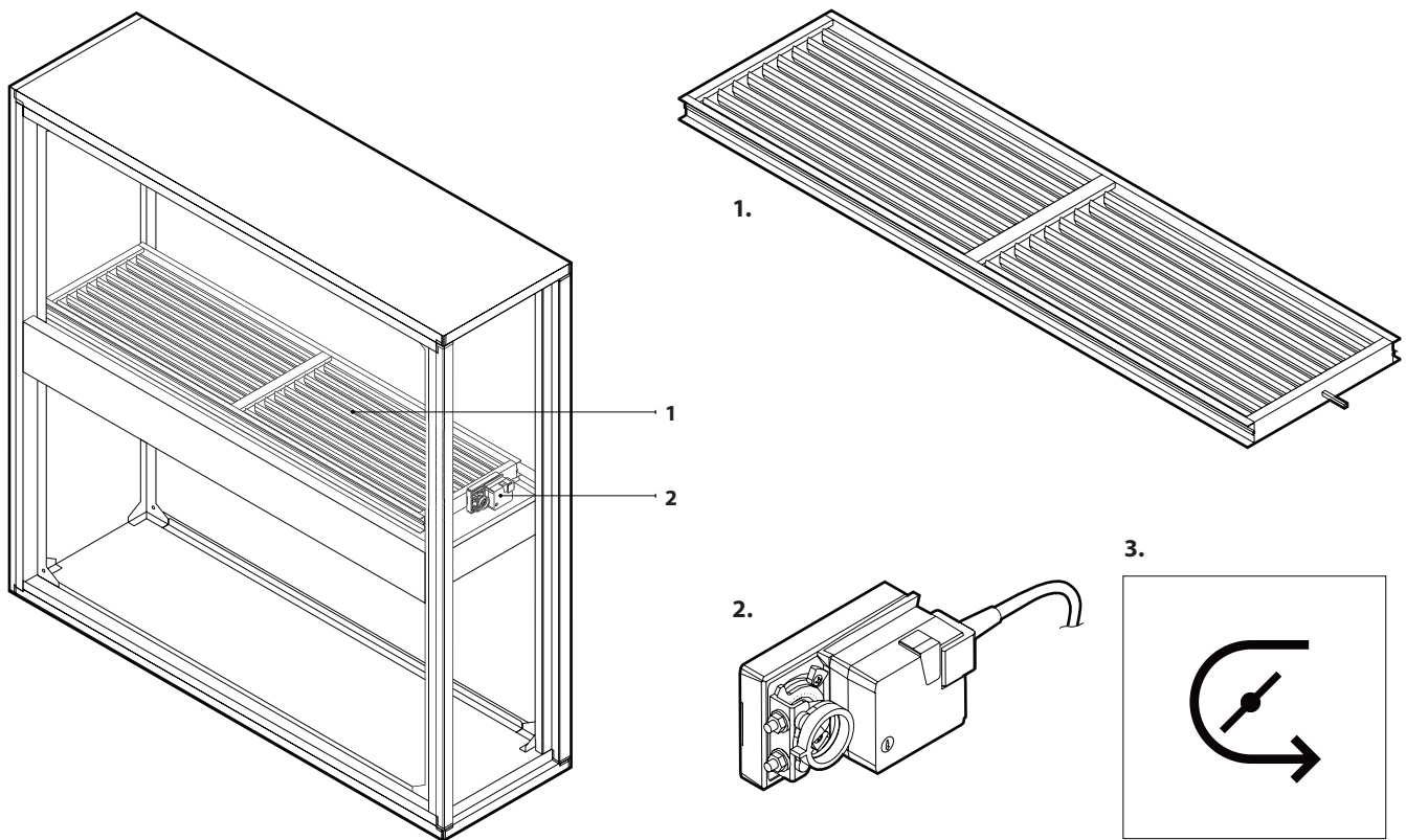
Fig. 4. Recirculatiesectie 1 – luchtmengklep, 2 – klepaandrijving, 3 – etiket recirculatiesectie
