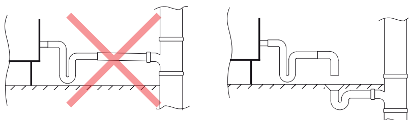
Fig. 23. Aansluiting van de condensaatafvoer op de riolering
