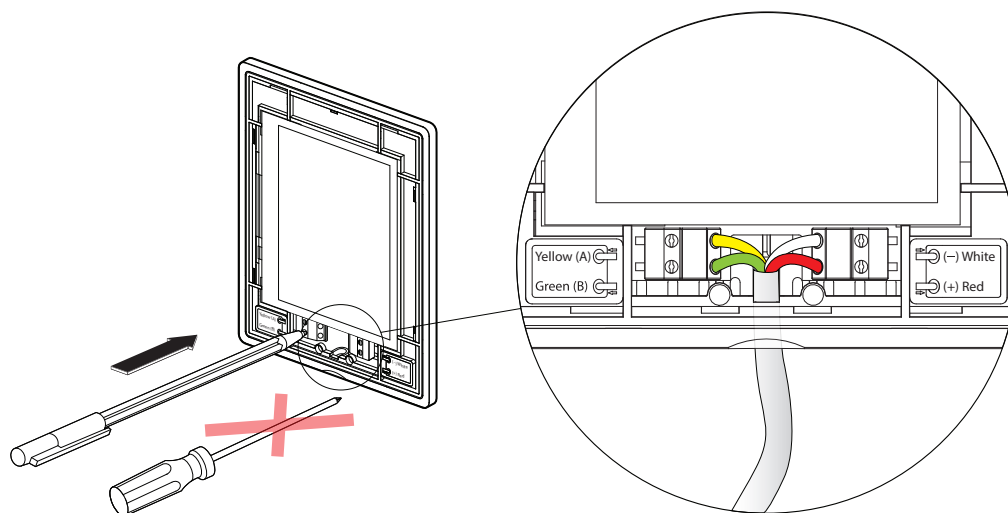
Fig. 38. Bedrading bedieningspaneel
