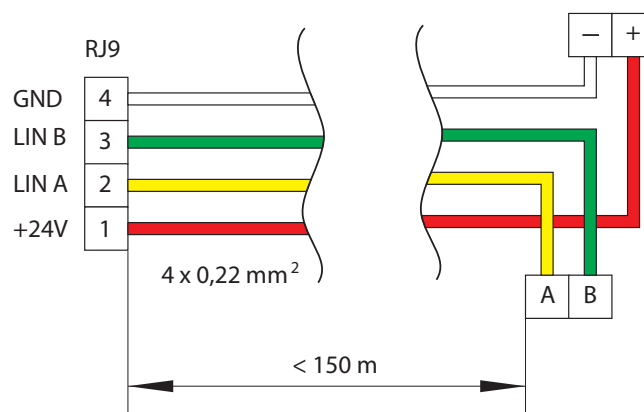
Fig. 37. Bedieningspaneel bedradingsschema
