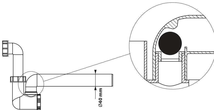
Fig. 22. Voorbeeld van een sifon met een eenrichtingsklep
