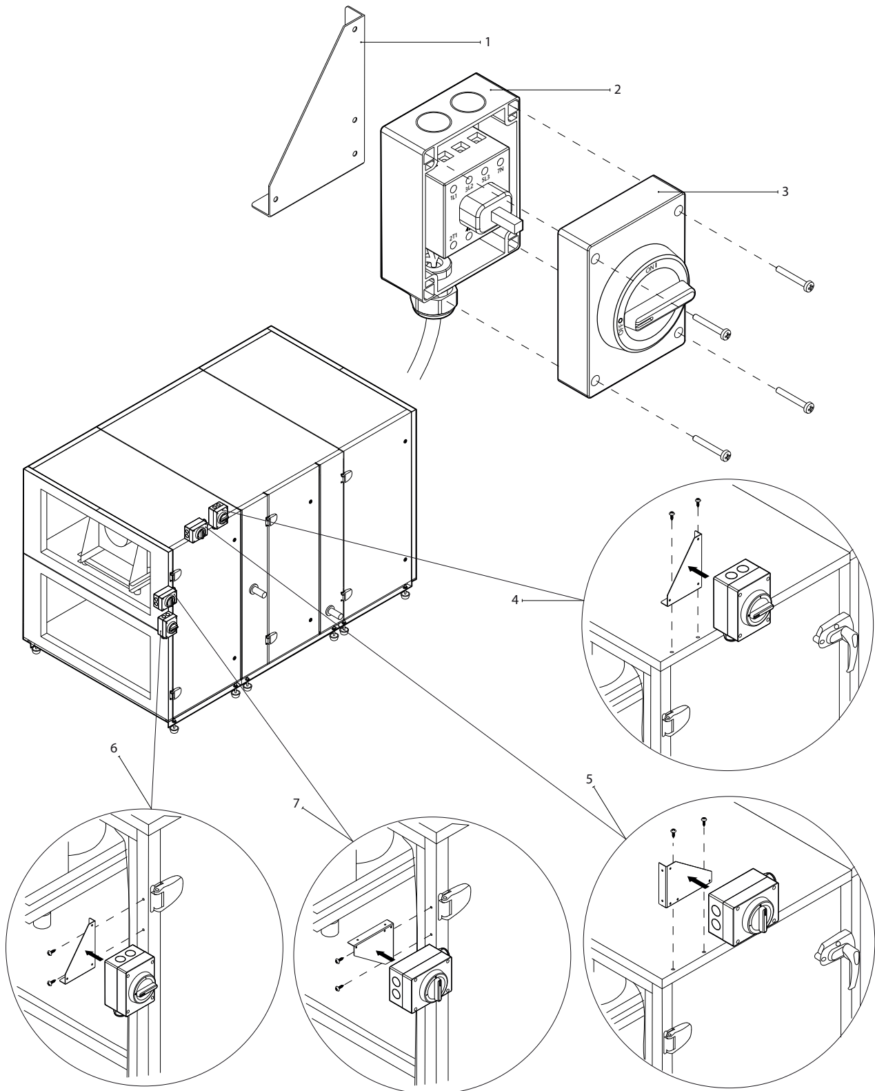
Fig. 28. Hoofdstroomonderbreker en montagevoorbeelden
