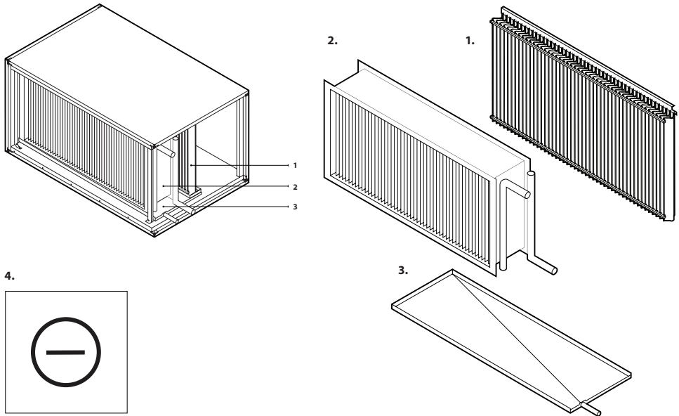
Fig. 6. Koelersectie
