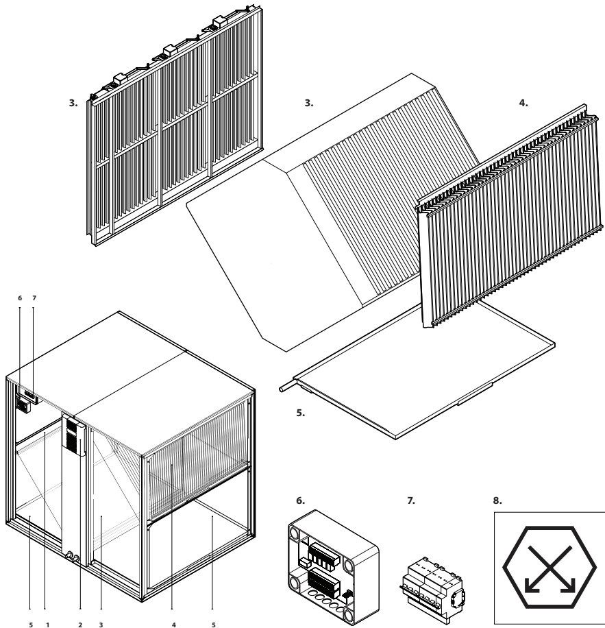
Fig. 2. Sectie Tegenstroomwarmtewisselaar (CF)
