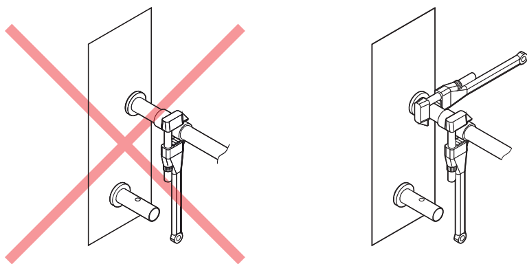
Fig. 25. Aansluiting van mouwen
