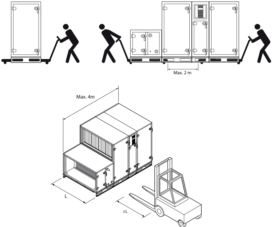
Fig. 13. Kastvervoer met behulp van een vorkheftruck of een trolley
