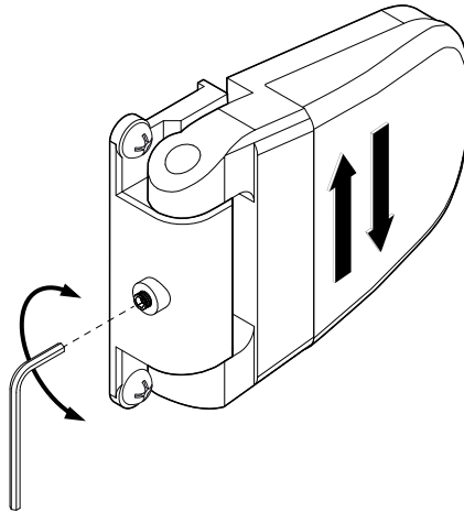
Fig. 20. Aanpassen van de scharnieren
