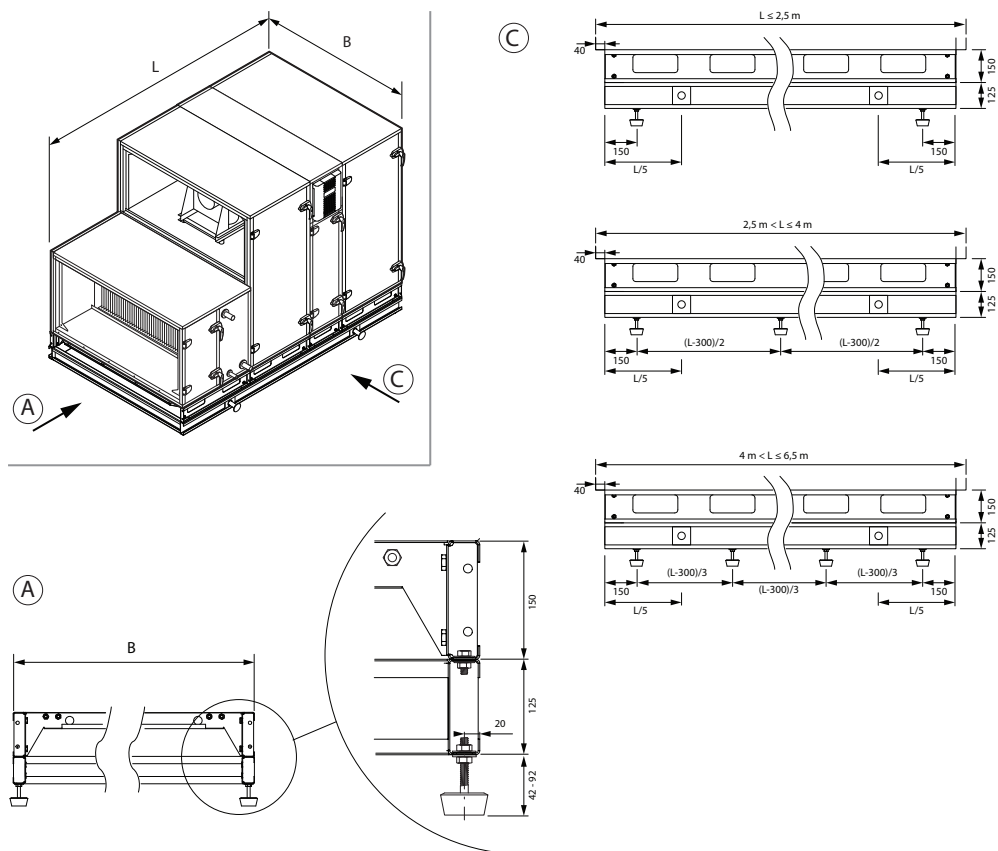
Fig. 16. Afmetingen van het versterkt montageframe
