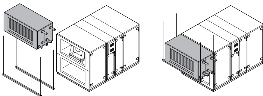
Fig. 24. Voorbeelden voor de installatie van verwarmings-/koelersecties
