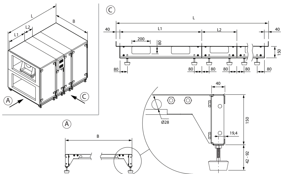
Fig. 17. Inbouwframe met verstelbare poten
