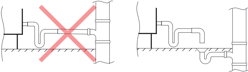
Fig. 30. Aansluiting van de condensaatafvoer op de riolering
