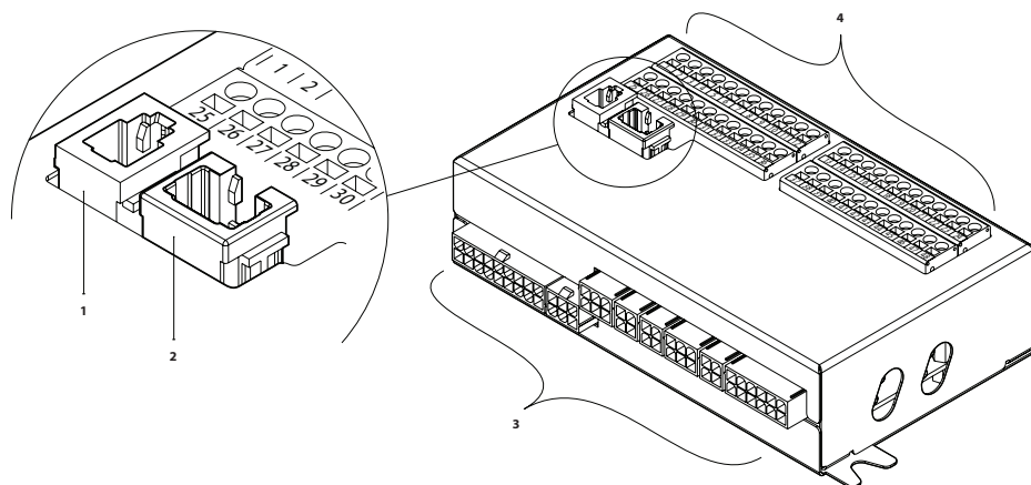
Fig. 38. Hoofdpaneel van het C5-bedieningspaneel
