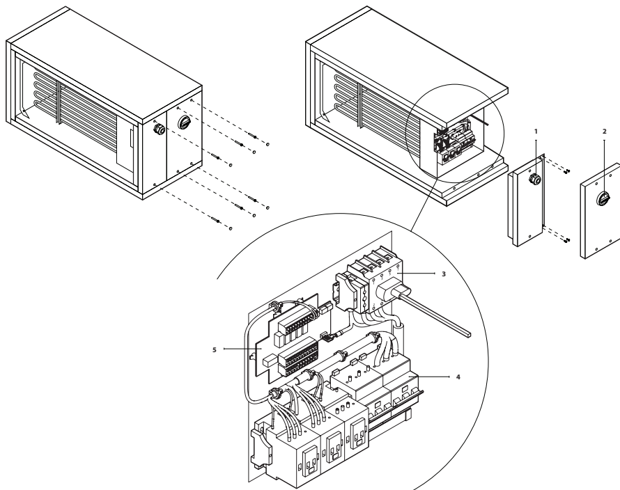
Fig. 36. Hoofdstroomonderbreker in een elektrisch verwarmingssectie
