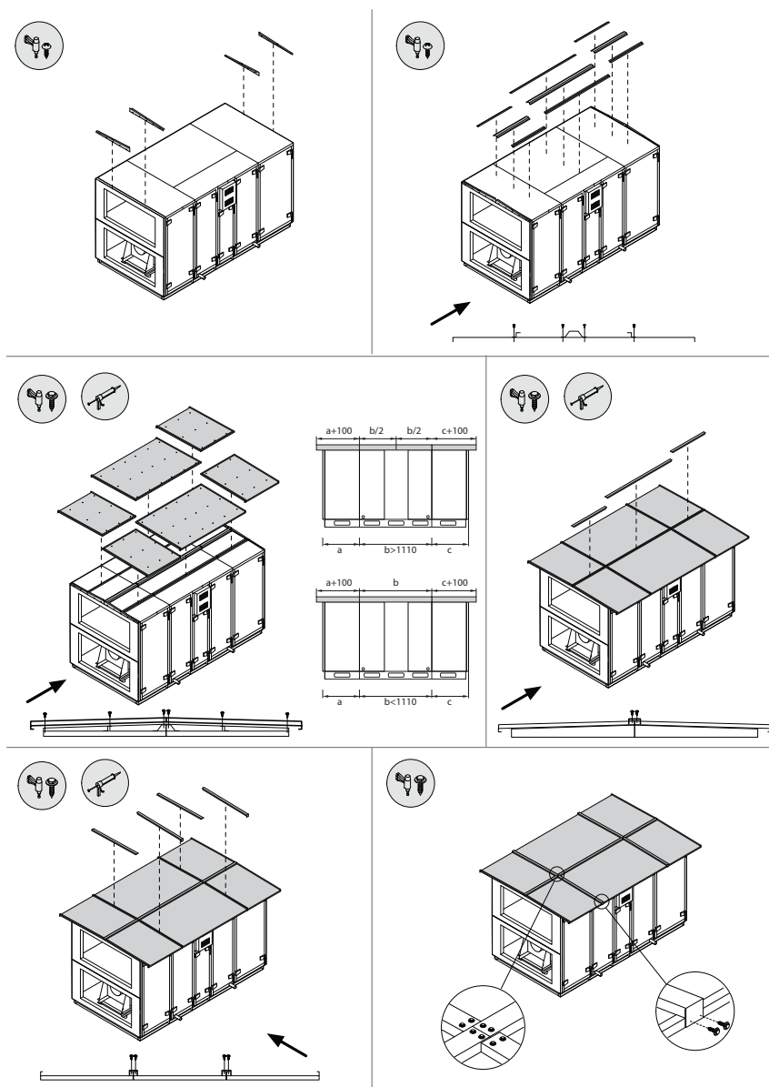
Fig. 34. Installatie van een afzonderlijk besteld beschermend dak 1
