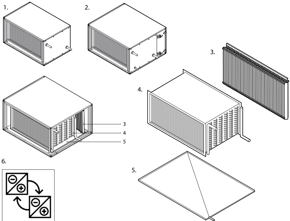
Fig. 4. Secties van vloeistofgekoppelde warmtewisselaar
