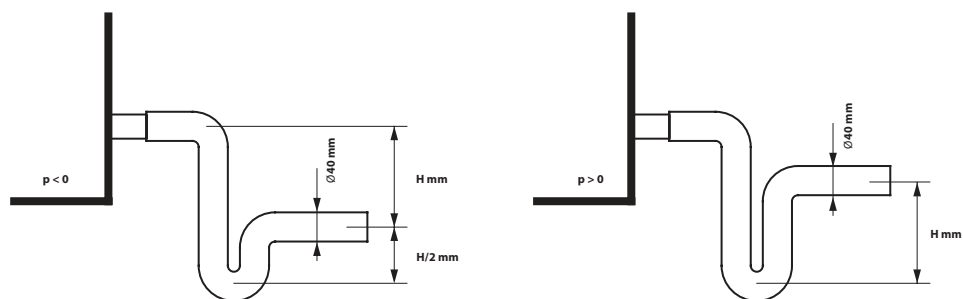
Fig. 28. Installatie van een sifon zonder eenrichtingsklep
