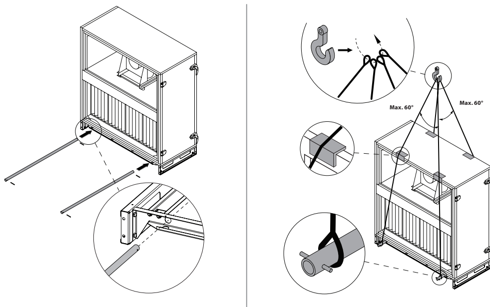
Fig. 14. Hijsen van afzonderlijke secties 1
