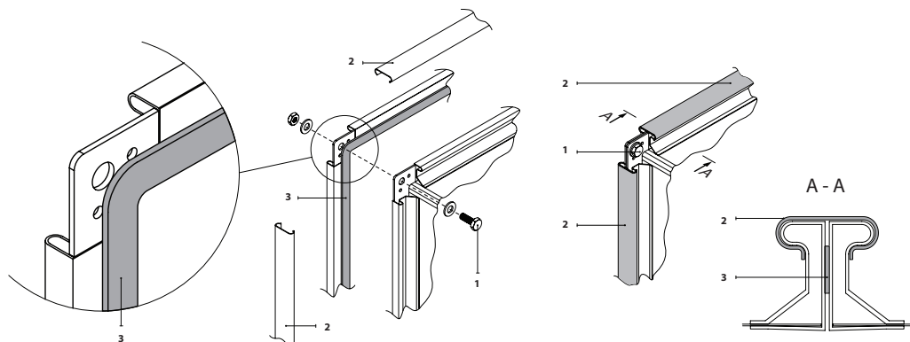
Fig. 31. Voorbeeld voor het bevestigen en afdichten van een flenskanaalverbinding 1 – schroef, 2 – C-profiel voor het aansluiten van flenzen, 3 – zelfklevende pakking
