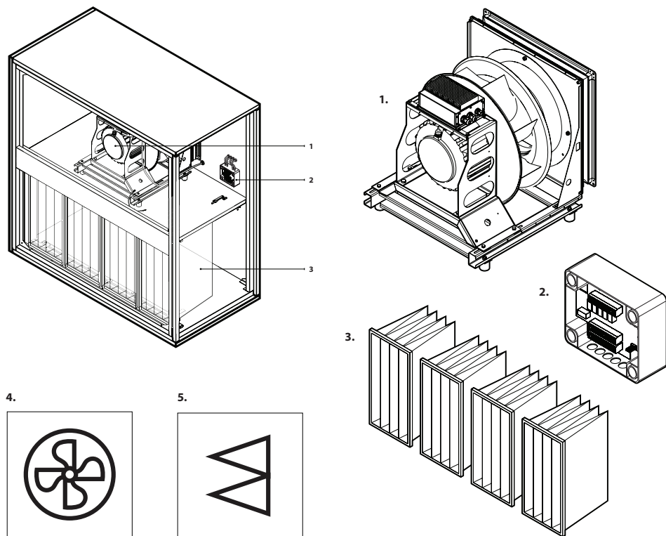
Fig. 1. Filterventilatorsectie
