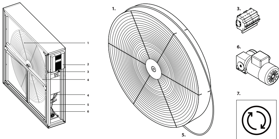
Fig. 3. Sectie Roterende Recuperator
