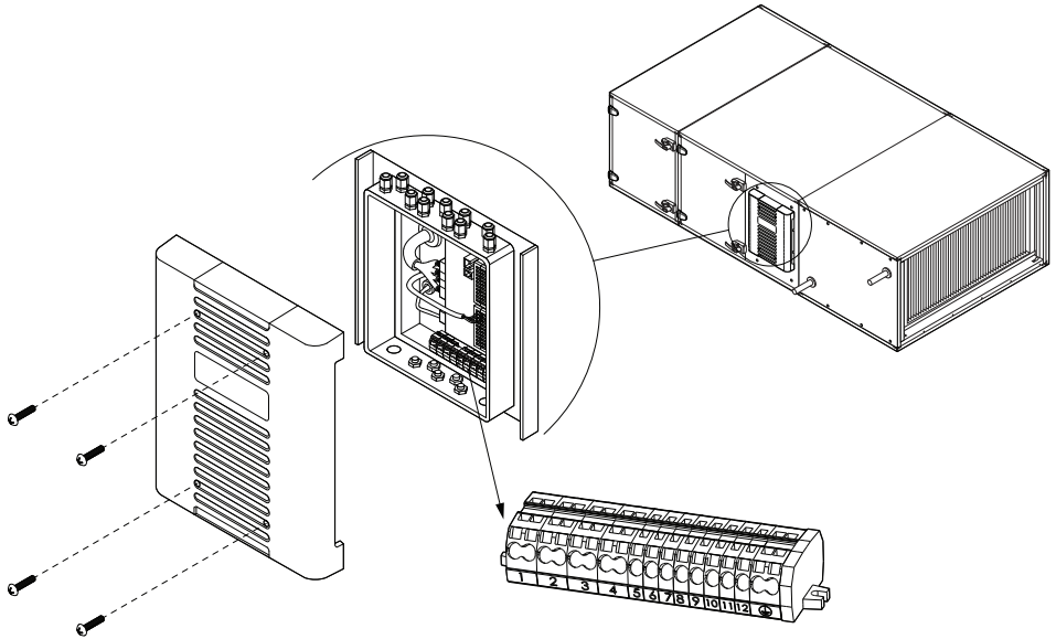
Fig. 46. Aansluitklemmen van VERSO RA luchtbehandelingskasten
