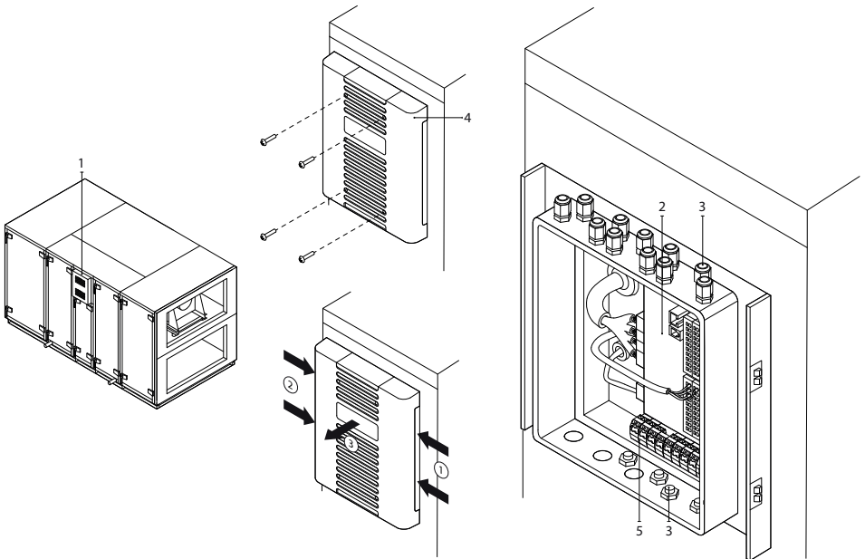
Fig. 37. Automatiseringskast
