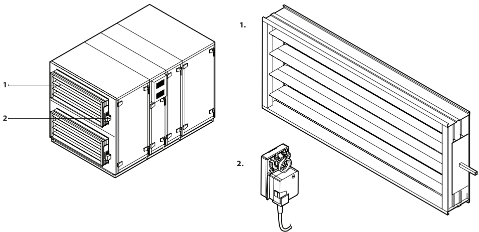
Fig. 8. Luchtafsluitende kleppen 1 – luchtklep, 2 – elektrische klepaandrijving
