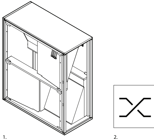
Fig. 12. Luchtstroomwisselingssectie 1 – luchtstroomwisselingssectie, 2 – sectie-etiket
