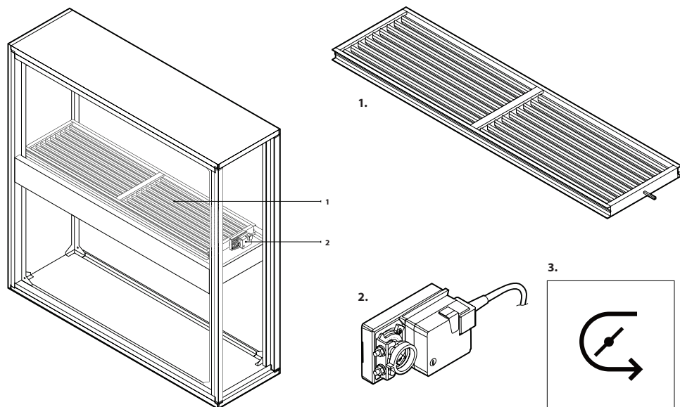
Fig. 5. Recirculatiesectie
