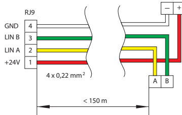
Fig. 48. Bedieningspaneel bedradingsschema
