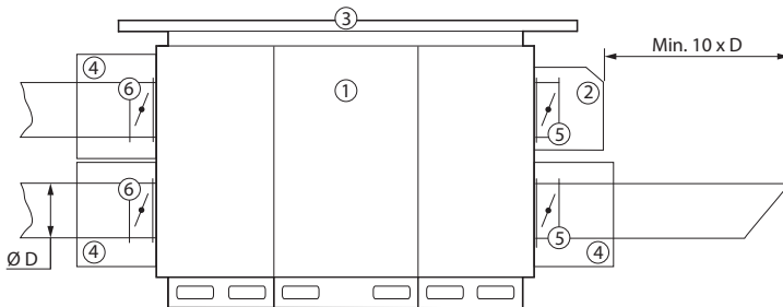
Afb. 33. Accessoires voor kasten die buiten worden geïnstalleerd
