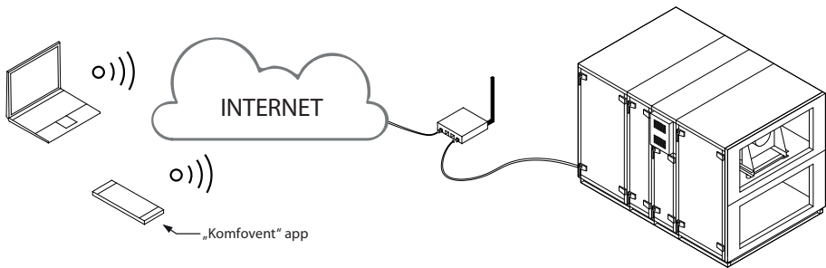
Fig. 54. Voorbeelden voor de LBK-verbinding met internet of het lokale netwerk
