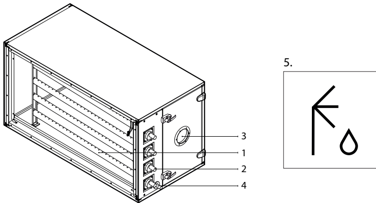
Fig. 10. Luchtbevochtiger
