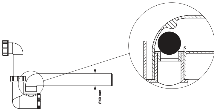
Fig. 29. Voorbeeld van een sifon met een eenrichtingsklep
