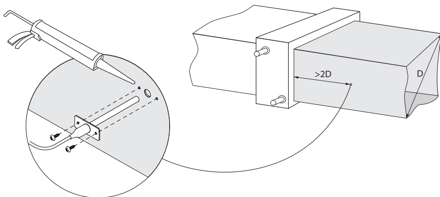
Fig. 43. Installatie van een toevoerluchttemperatuursensor
