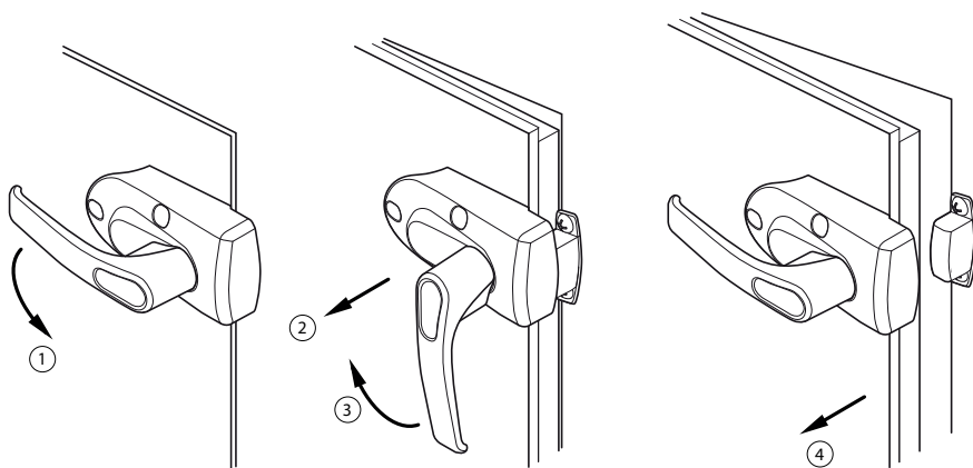
Fig. 19. Het openen van de deur
