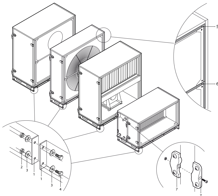
Fig. 21. Externe aansluiting en afdichting van secties
