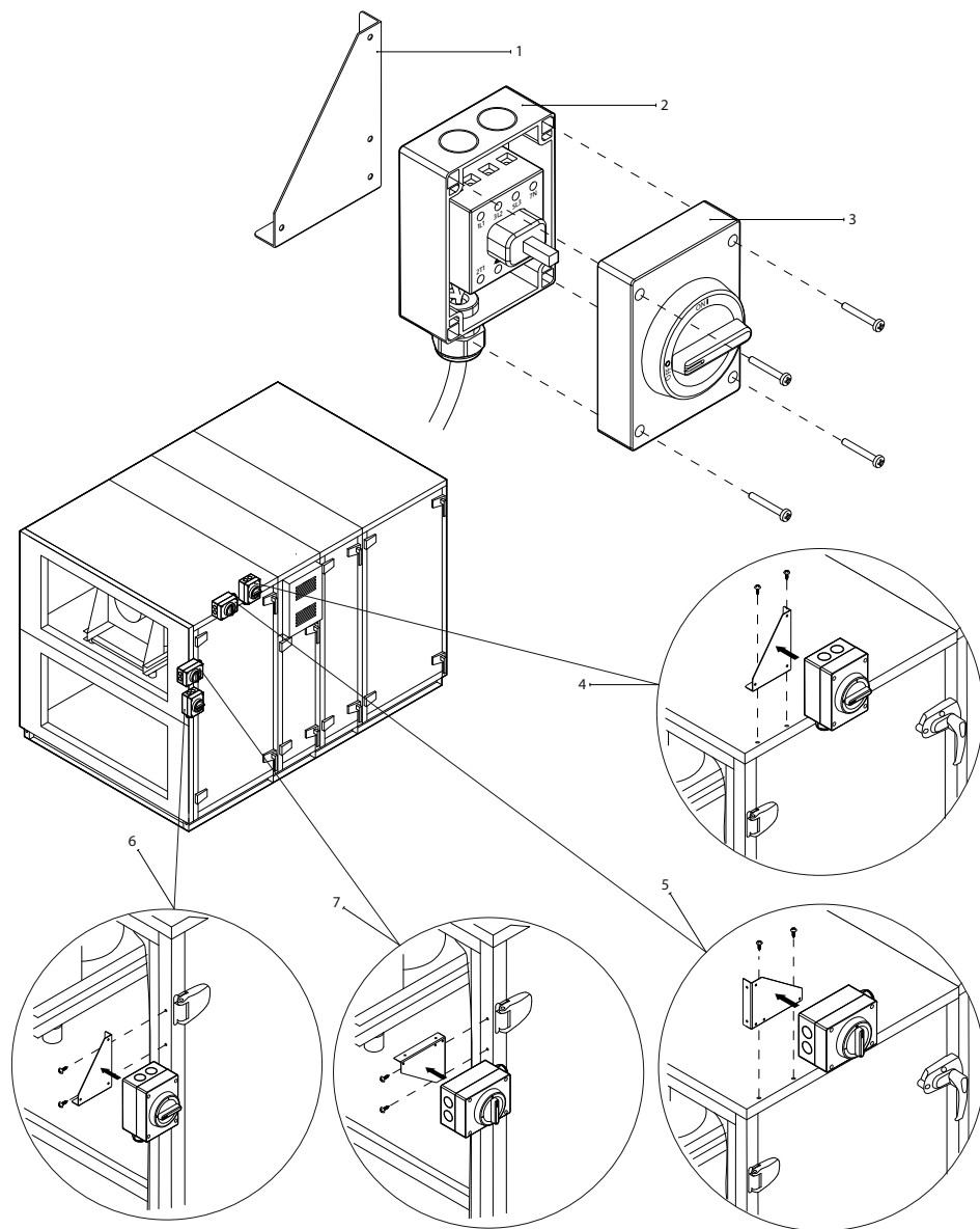
Fig. 35. Hoofdstroomonderbreker en montagevoorbeelden
