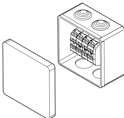
Fig. 51. Aftakdoos PD1
