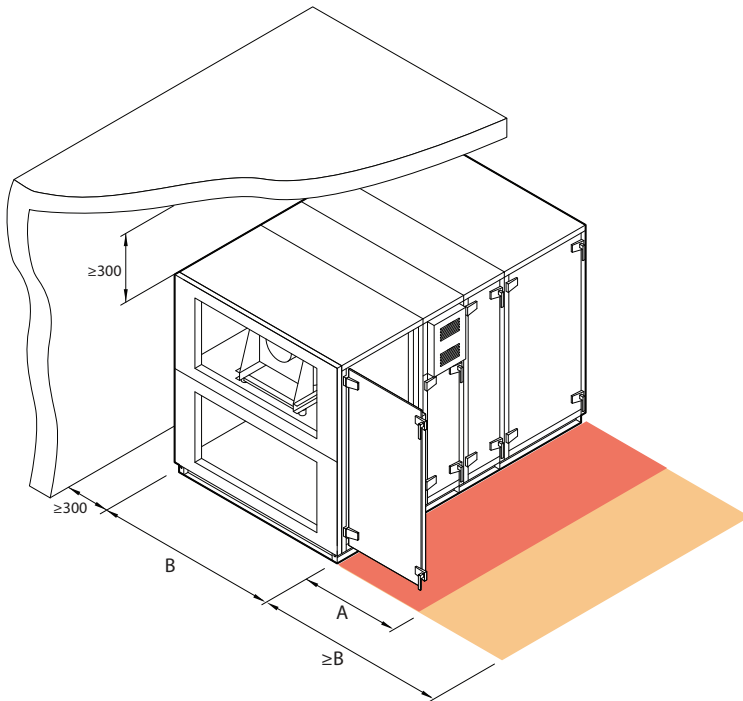
Fig. 18. Kastinspectiegebied
