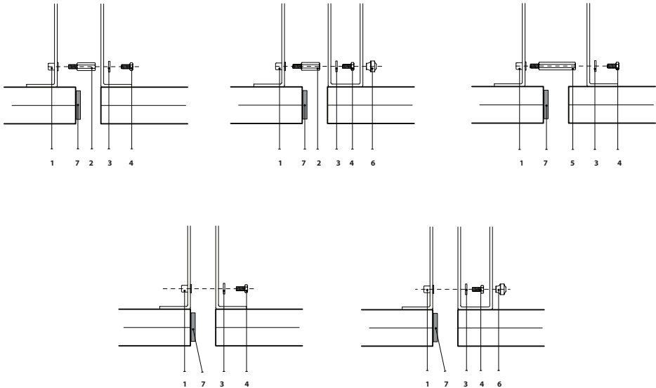
Fig. 22. Soorten interne sectieverbindingen
