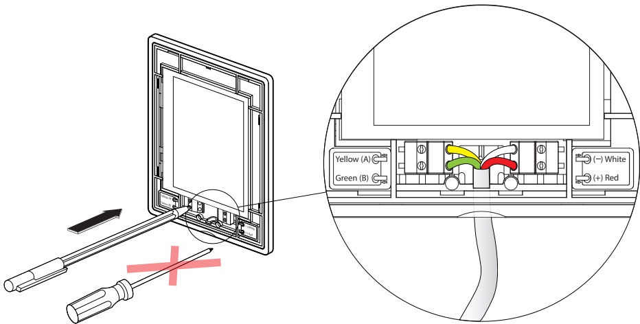
Fig. 49. Bedrading bedieningspaneel
