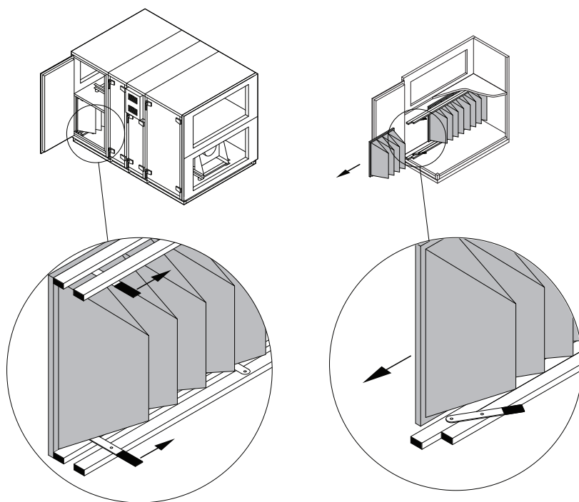
Fig. 55. Filterkleminrichting
