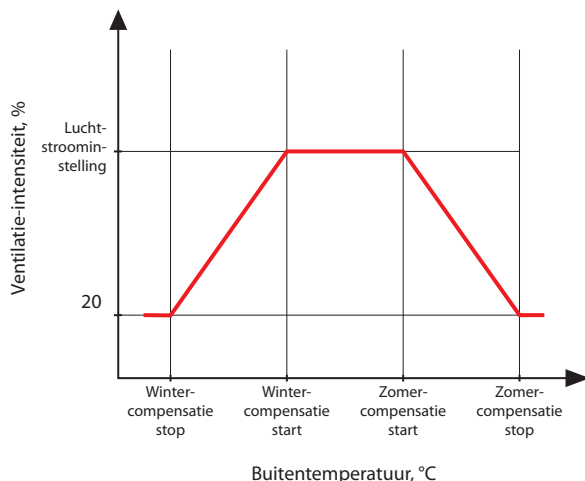
Fig. 1. OCV-functiebediening
