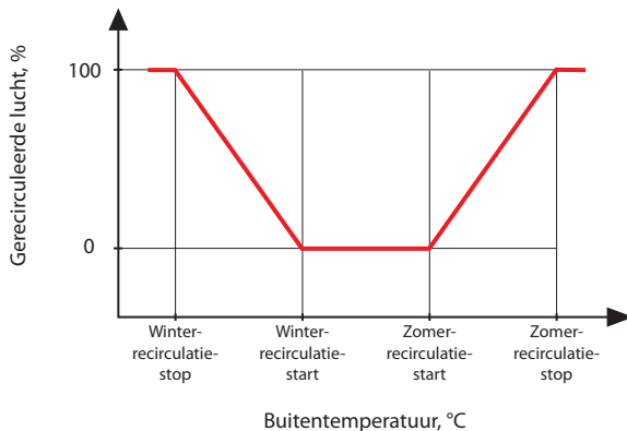
Fig. 2. REC-functiebediening
