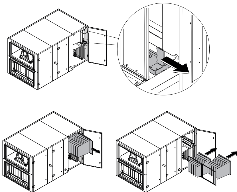
Fig. 3. Filterkleminrichting
