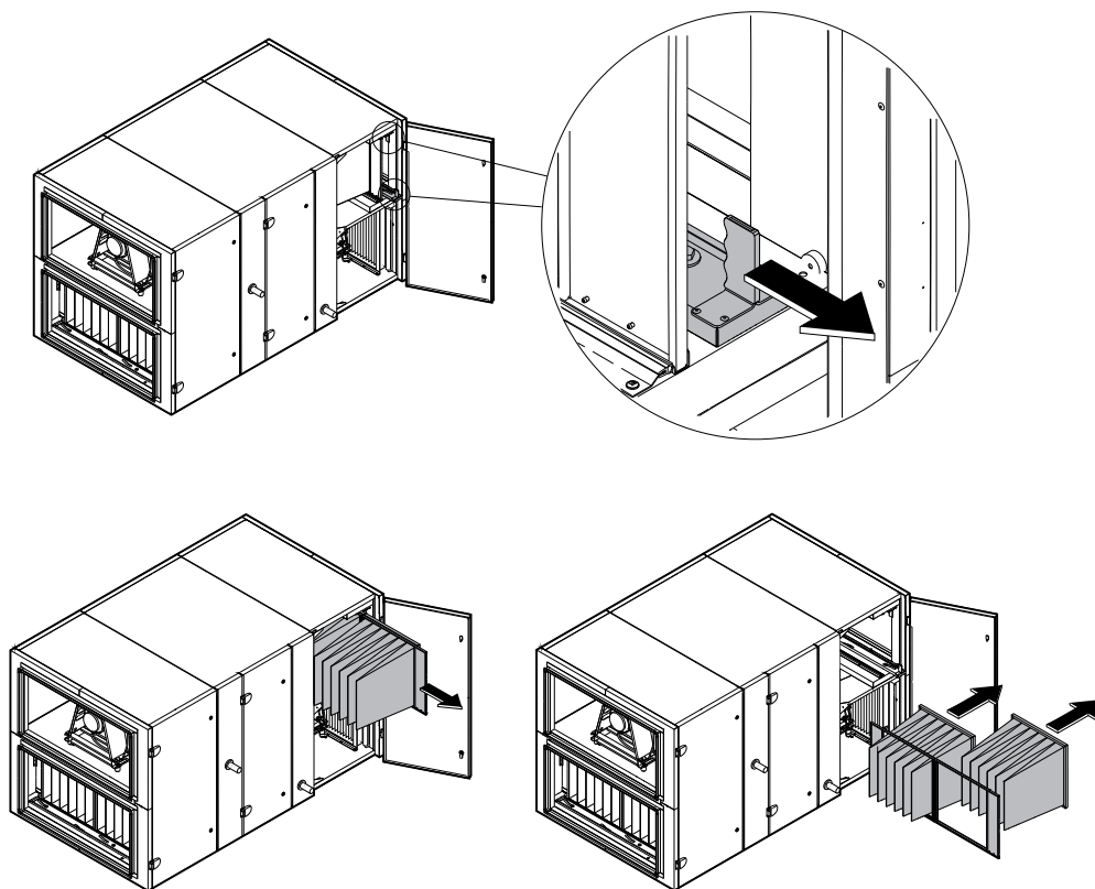
Fig. 46. Filterkleminrichting
