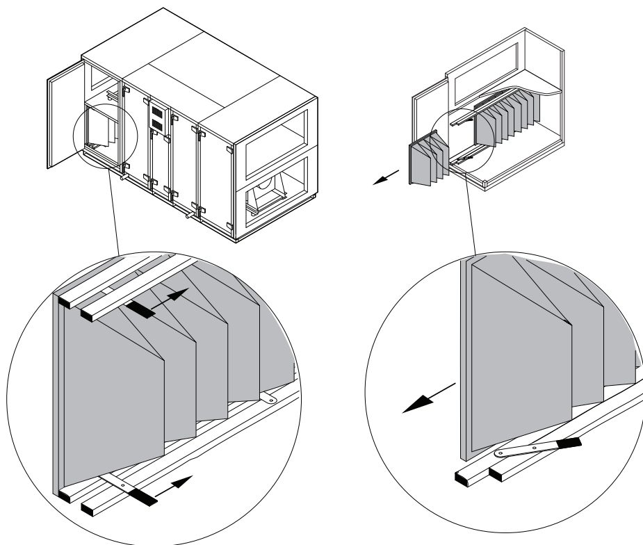
Fig. 3. Filterkleminrichting
