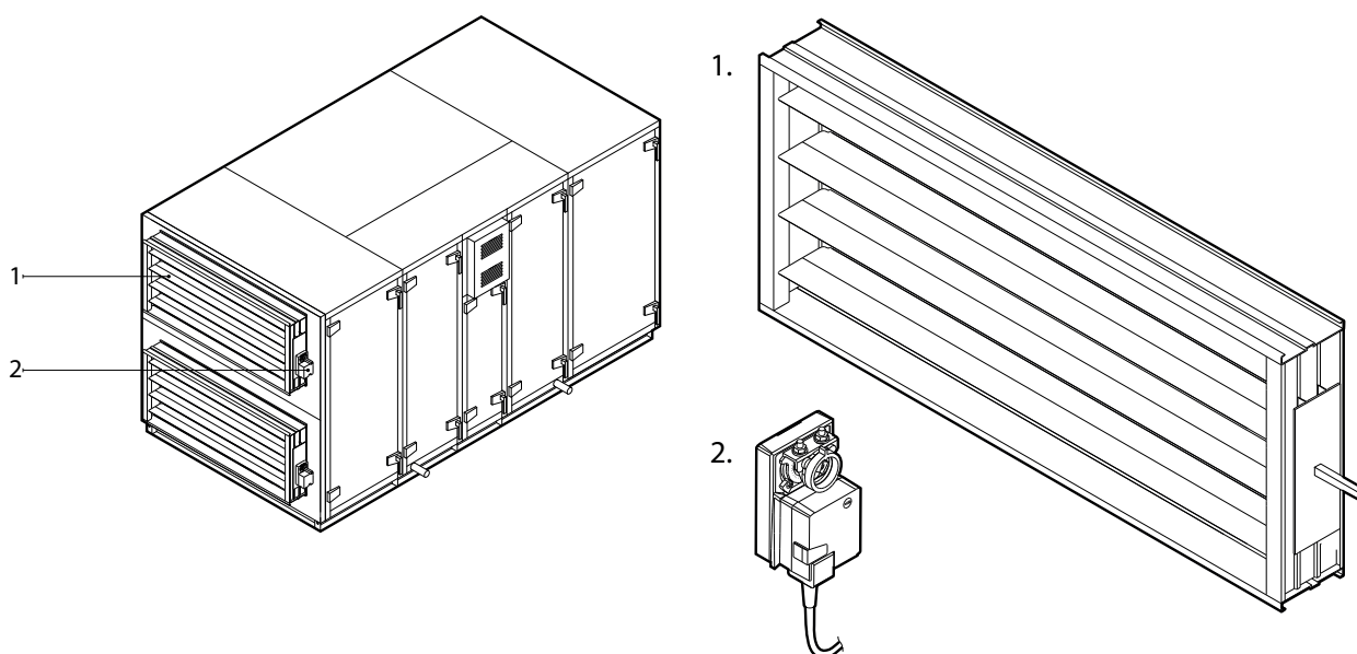
Fig. 9. Luchtafsluitende kleppen
