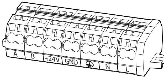
Fig. 44. Extra aansluitklemmenblok
