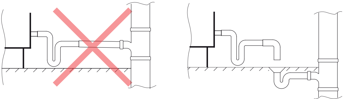
Fig. 30. Aansluiting van de condensatafvoer op de riolering
