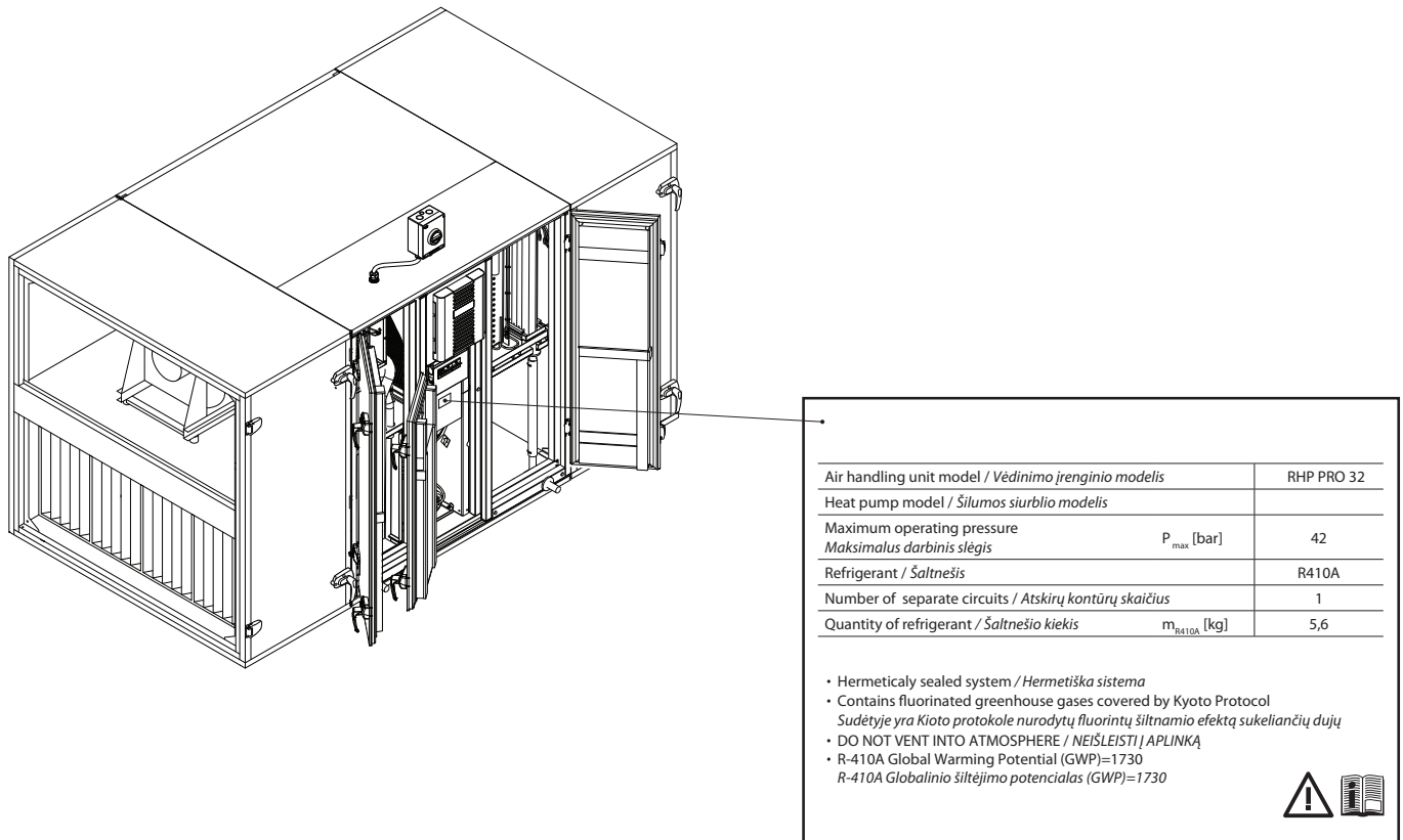
Fig. 5. Voorbeeld van het informatie-etiket van een warmtepomp
