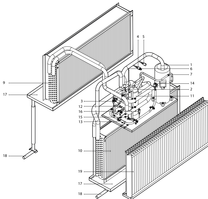
Fig. 4. Hydraulisch schakelschema en onderdelen van de warmtepomp
