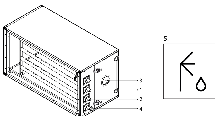
Fig. 11. Luchtbevochtiger
