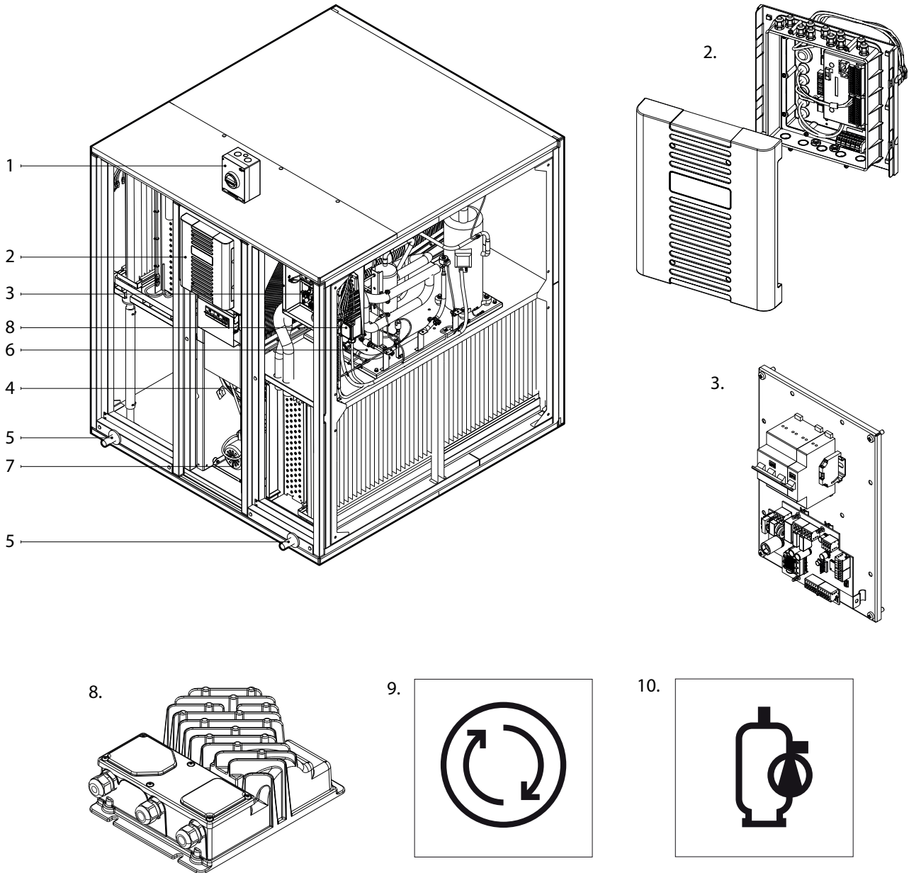
Fig. 2. Warmtepompsectie
