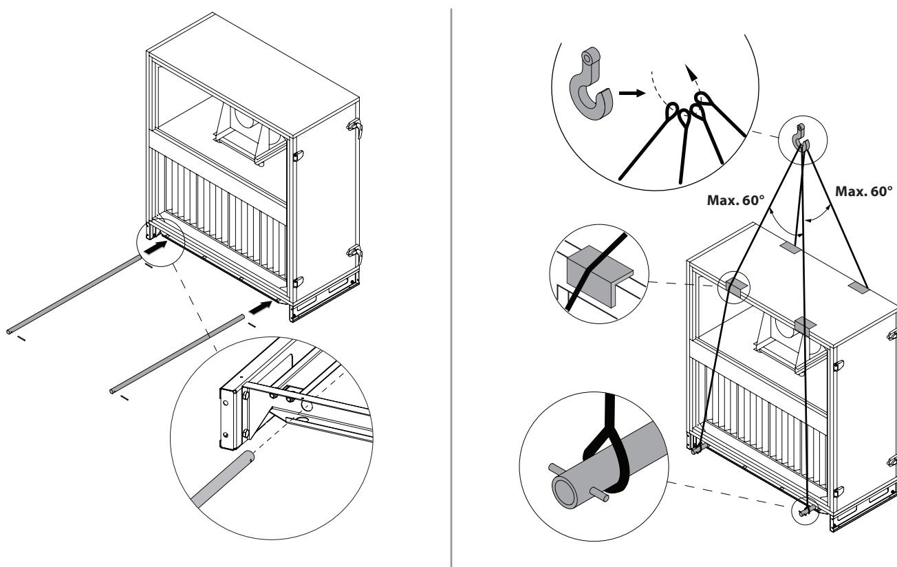
Fig. 14. Hijsen van afzonderlijke secties 1
