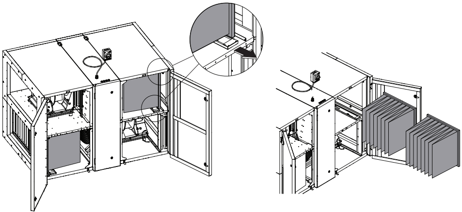
Afb. 31. Een voorbeeld van het vervangen van zakkenfilters
