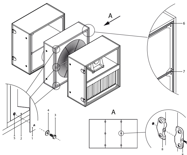
Afb. 11. Aansluiting van secties en hun afdichting
