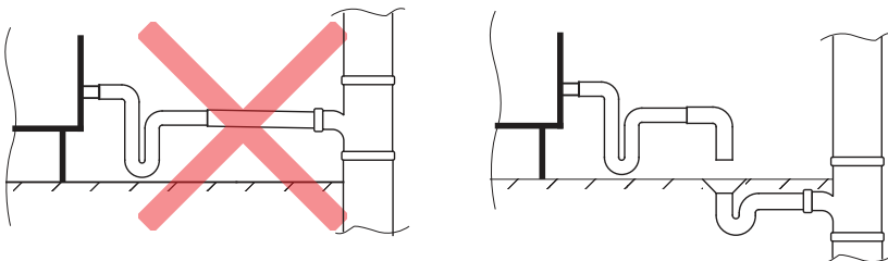
Afb. 17. Aansluiting van de condensafvoer op de riolering
