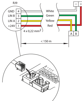
Afb. 24. Bedieningspaneel bedradingsschema
