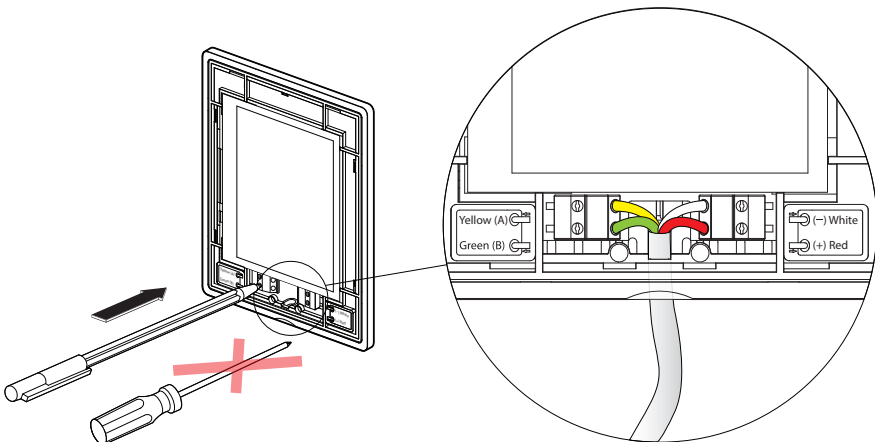
Afb. 25. Bedrading bedieningspaneel
