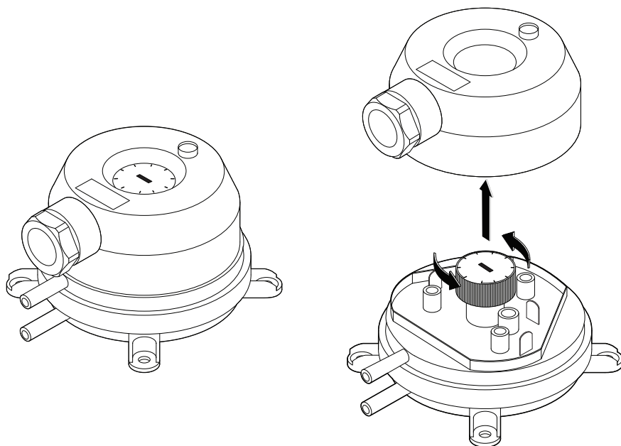
Afb. 30. Drukschakelaar
