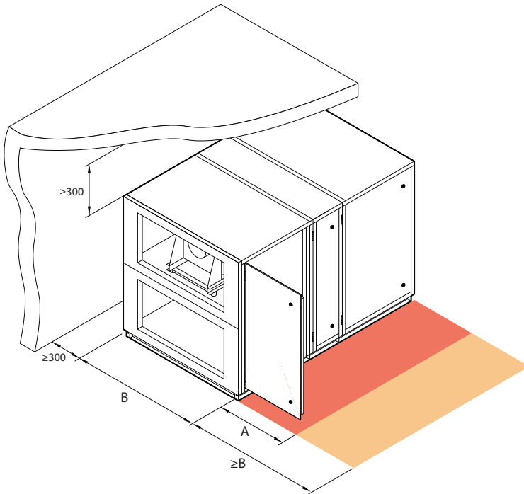
Afb. 9. Kastinspectiegebied
