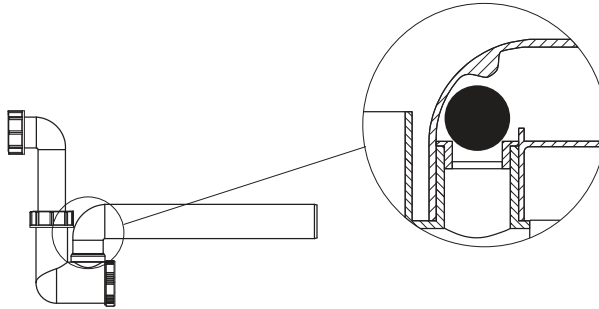
Afb. 16. Voorbeeld van een sifon met een eenrichtingsklep
