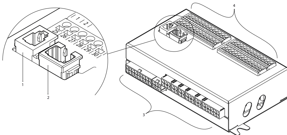
Afb. 19. C5-regeling hoofdpaneel
