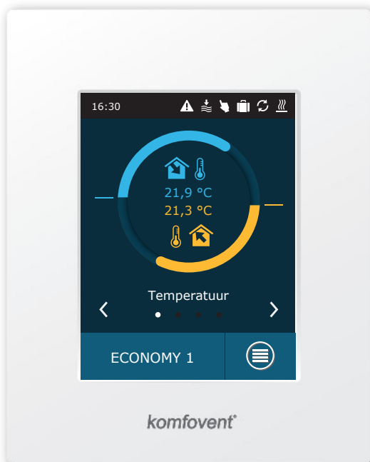
Afb. 32. Bedieningspaneel
