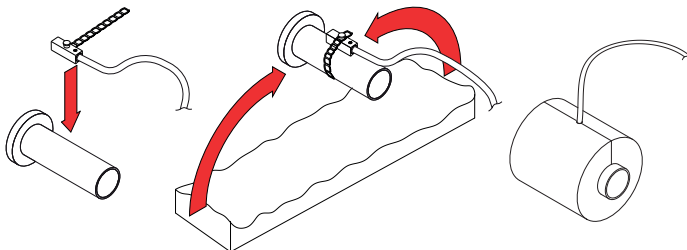
Afb. 14. Installatie van een retourwatertemperatuursensor
