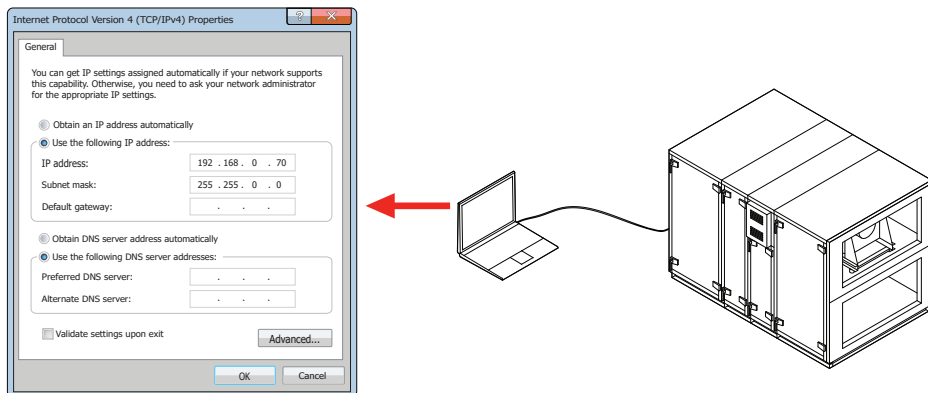
Afb. 28. Computernetwerkinstellingen voor directe aansluiting op de kast
