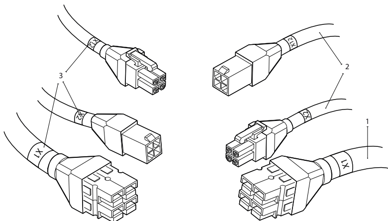
Afb. 26. Kabelverbindingen tussen secties
