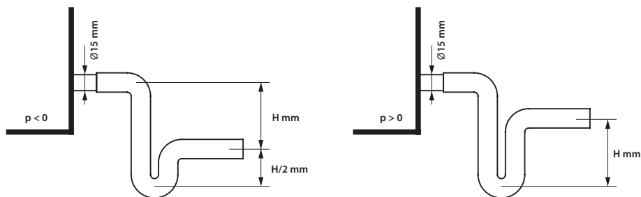
Afb. 15. Installatie van een sifon
