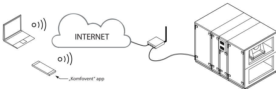
Afb. 29. Voorbeelden voor de LBK-verbinding met internet of het lokale netwerk
