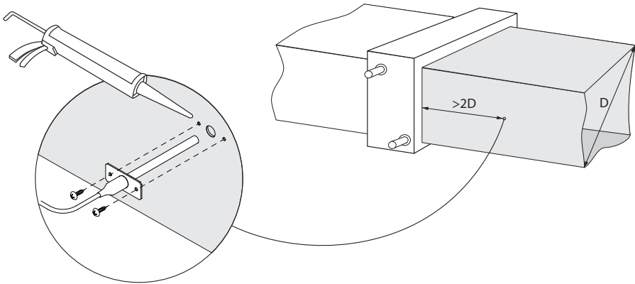
Afb. 23. Installatie van een toevoerluchttemperatuursensor
