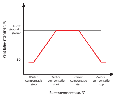
Fig. 1. OCV-functiebediening
