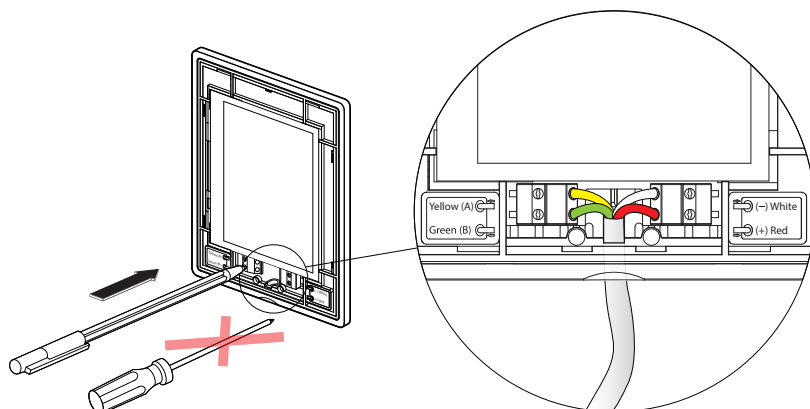
Afb. 20. Bedrading bedieningspaneel
