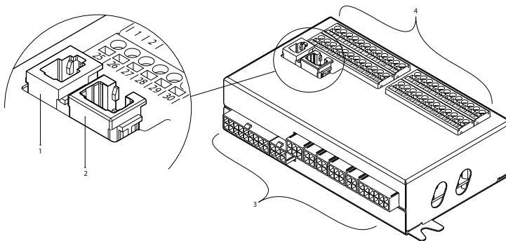
Afb. 14. C5-regeling hoofdpaneel
