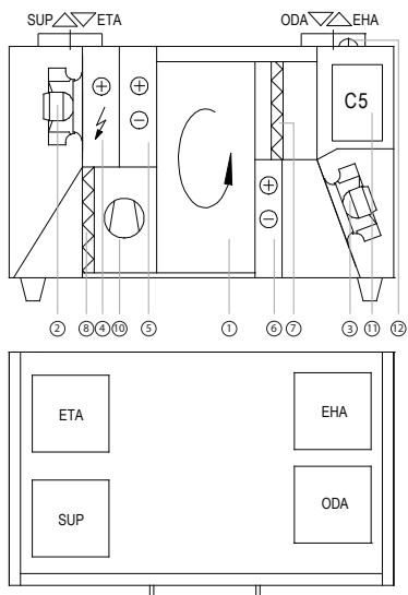
Linker inspectiezijde L1
