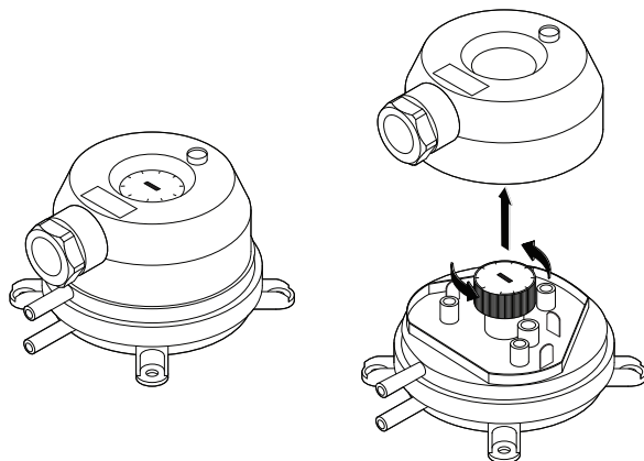
Afb. 24. Drukschakelaar
