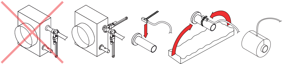
Afb. 9. Het aansluiten van de waterslangen op de verwarming/koeler en het installeren van de watertemperatuursensor
