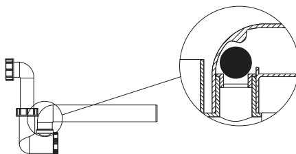
Afb. 11. Voorbeeld van een sifon met een eenrichtingsklep
