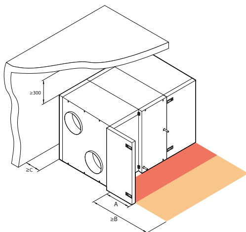
Afb. 8. Kastinspectiegebied
