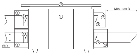
Afb. 13. Accessoires voor kasten die buiten worden geïnstalleerd
