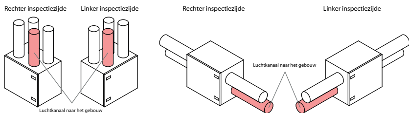
Afb. 6. Indeling van kasten o.b.v. de inspectiezijde
