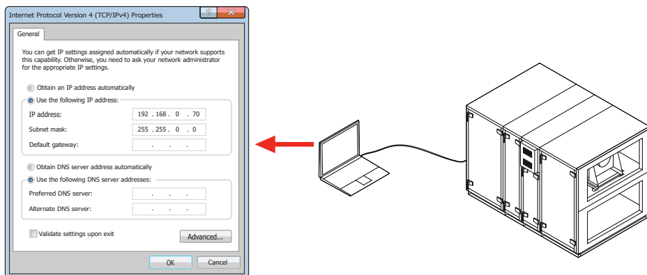
Afb. 22. Computernetwerkinstellingen voor directe aansluiting op de kast
