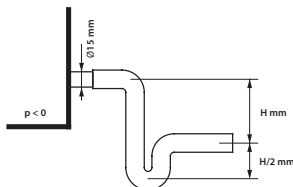
Afb. 10. Installatie van een sifon
