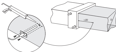
Afb. 18. Installatie van een toevoerluchttemperatuursensor
