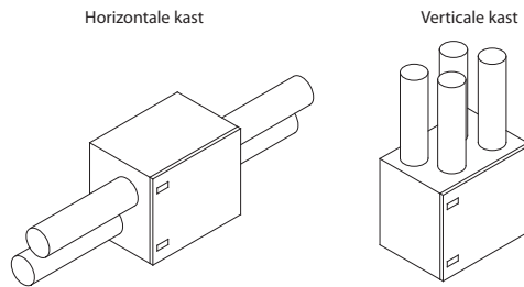
Afb. 4. Classificatie van kasten o.b.v. het type kanaalaansluiting
