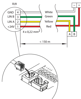
Afb. 19. Bedieningspaneel bedradingsschema
