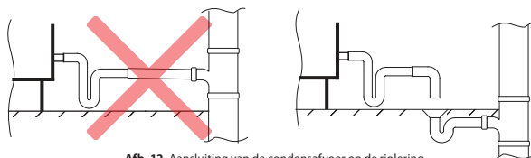
Afb. 12. Aansluiting van de condensafvoer op de riolering
